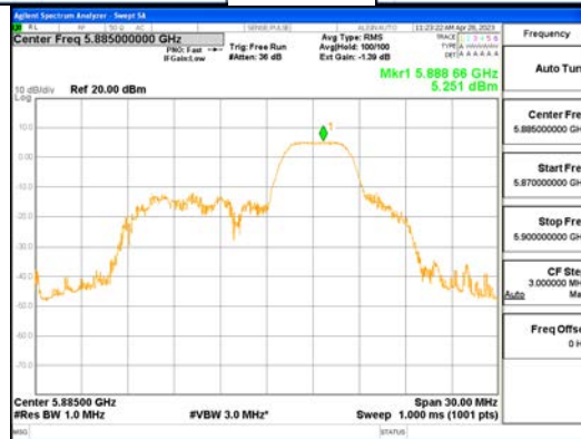
ANTO_802.11ax_HE20_52T_Mid_UNI I 4
