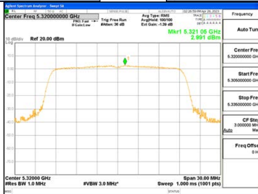
ANTO_802.11ax_HE20_242T_UNII 2A
