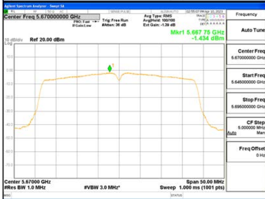
ANTO_802.11ac_VHT40_UNII 2C
