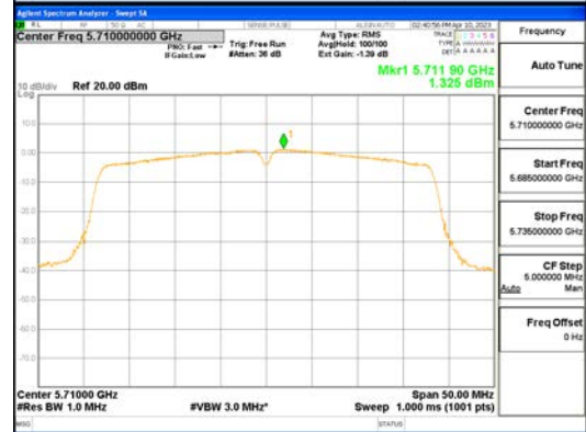
ANTO_802.11n_HT40_UNII 2C
