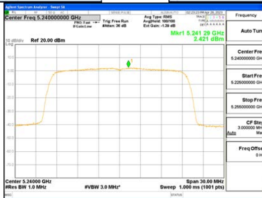
ANTO_802.11ax_HE20_242T_UNII 1
