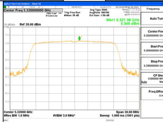
ANT1_802.11ax_HE20_242T_UNII 2A
