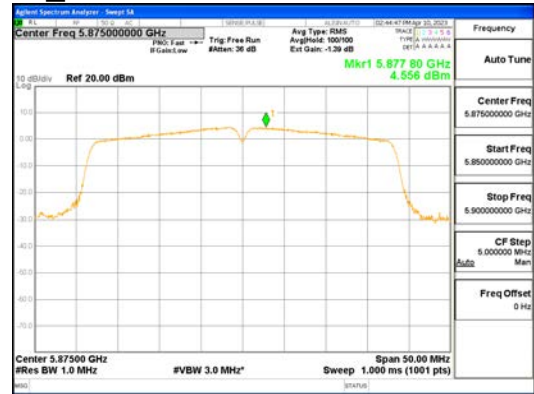
ANTO_802.11n_HT40_UNI I 4
