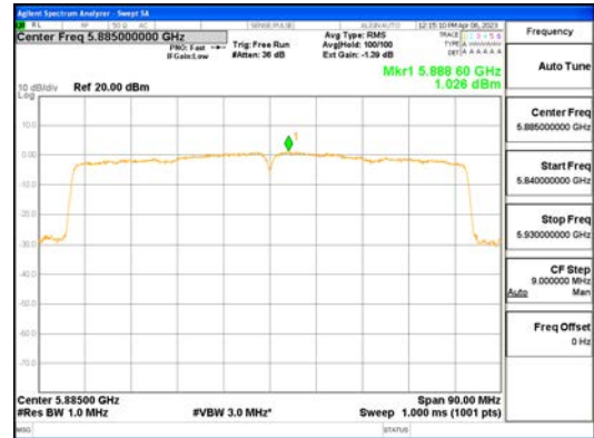
ANTO_802.11ac_VHT80_UNII 4
