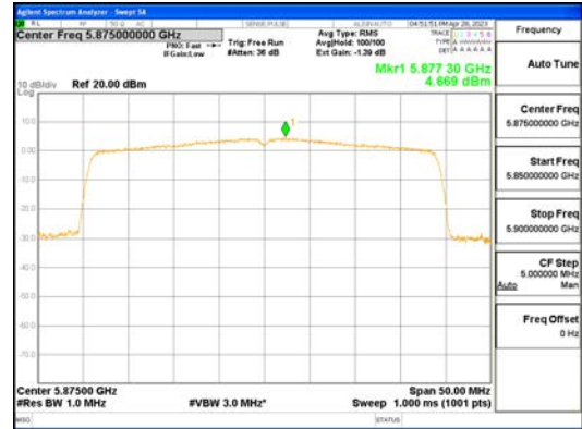
ANTO_802.11ax_HE40_484T_UNI 4
