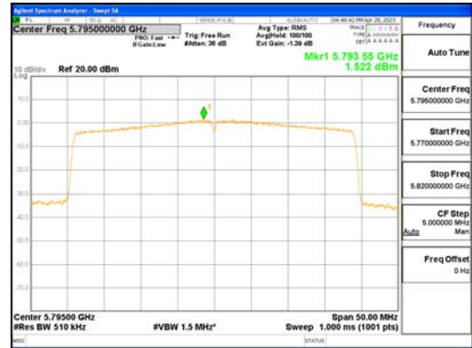
ANTO_802.11ax_HE40_484T_UNI 3
