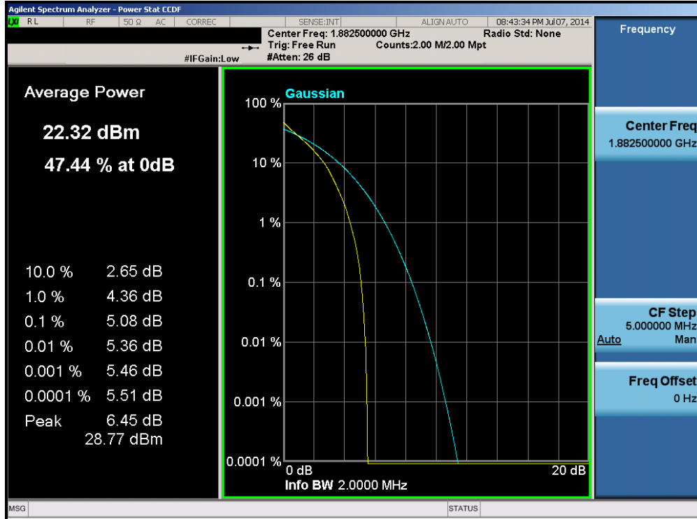
Plot 6-97. PAR Plot (Band 25 – 1.4MHz QPSK – RB Size 6)
