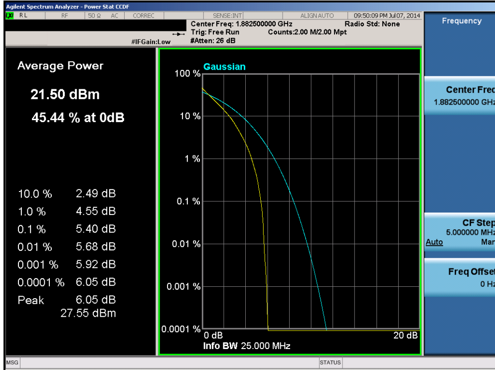
Plot 6-99. PAR Plot (Band 25 – 15.0MHz QPSK – RB Size 75)
