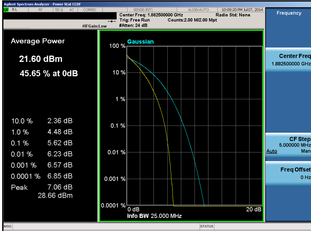
Plot 6-101. PAR Plot (Band 25 – 20.0MHz QPSK – RB Size 100)
