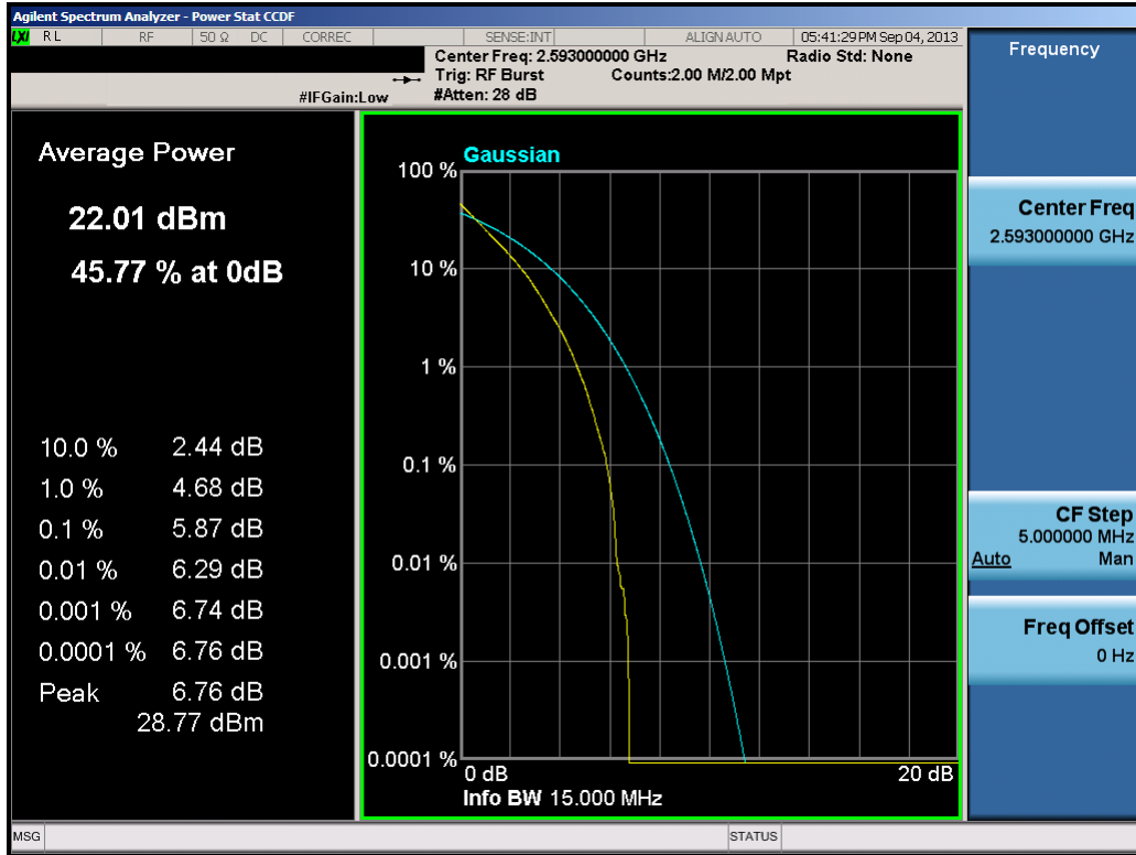
Plot 9-20. PAR Plot (15.0MHz QPSK – RB Size 75)
