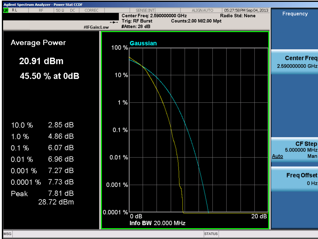
Plot 9-30. PAR Plot (20.0MHz 16-QAM – RB Size 100)
