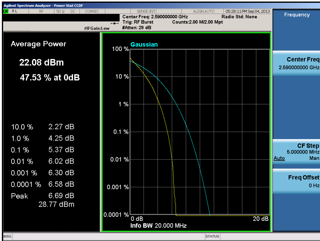
Plot 9-29. PAR Plot (20.0MHz QPSK – RB Size 100)
