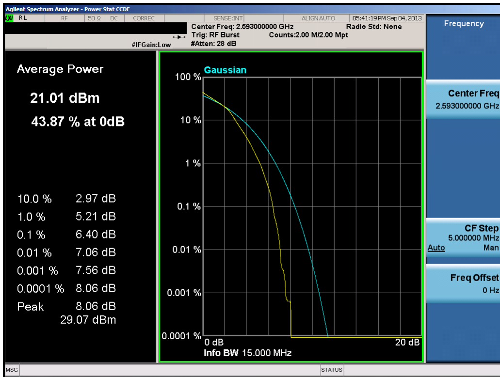
Plot 9-21. PAR Plot (15.0MHz 16-QAM – RB Size 75)
