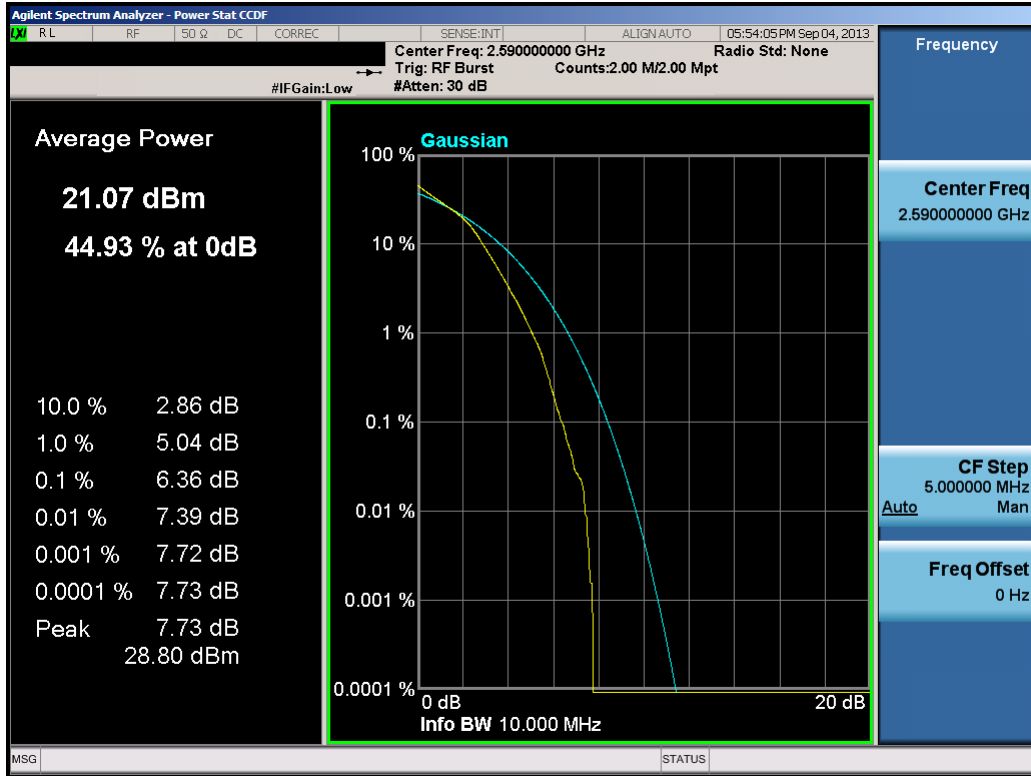
Plot 9-6. PAR Plot (10.0MHz 16-QAM – RB Size 50)
