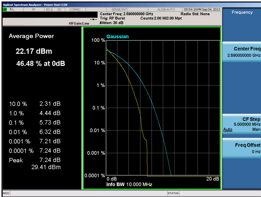
Plot 9-5. PAR Plot (10.0MHz QPSK – RB Size 50)
