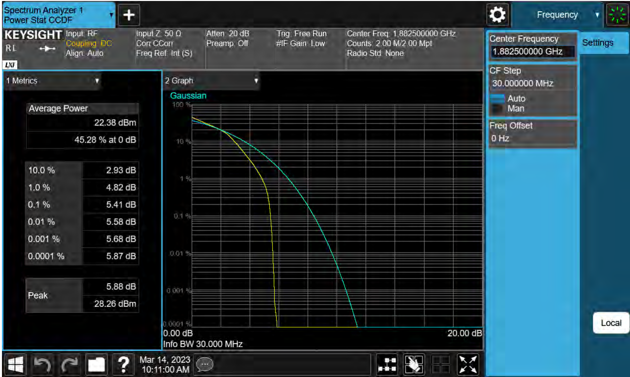
Sub6 n25. PAR Plot (30 M BW Ch.376500 16QAM_ Full RB_0)
