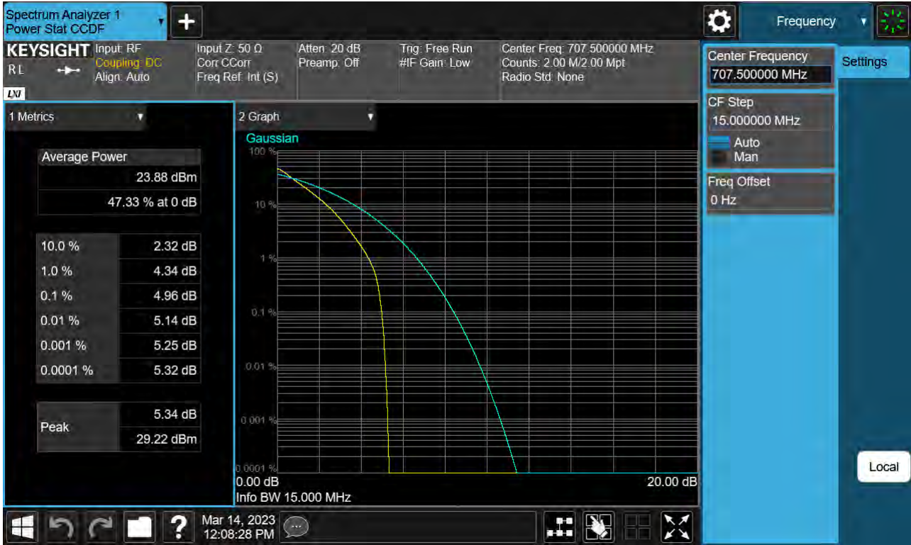
Sub6 n12. PAR Plot (15M BW Ch.141500 QPSK_RB75_0)
