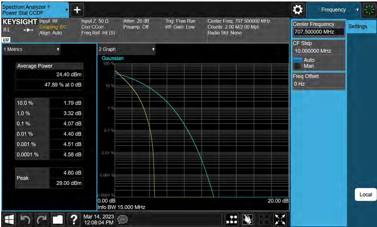
Sub6 n12. PAR Plot (15M BW Ch.141500 BPSK_RB75_0)
