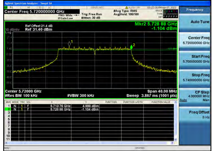
802.11n_HT20 CH.144
