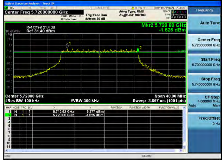
802.11n_HT20 CH.144
