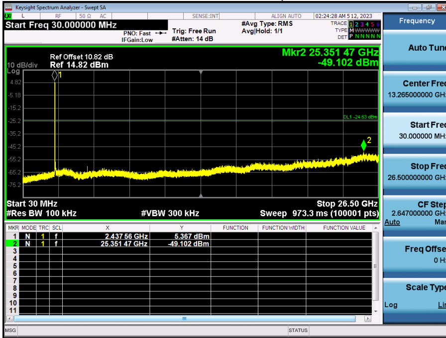
802.11b_Ch.6_1 Mbps
