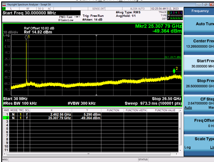
802.11b_Ch.11_1 Mbps
