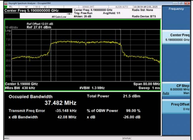
Bandwidth 40M Ch.38(5190 MHz) SU
