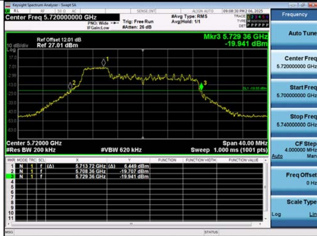
40M Ch.142(5710 MHz) SU
