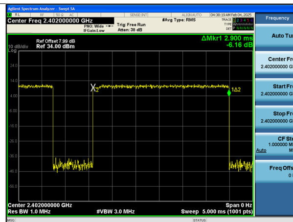
\pi/4 DQPSK : Dwell Time(Ch. 0)
