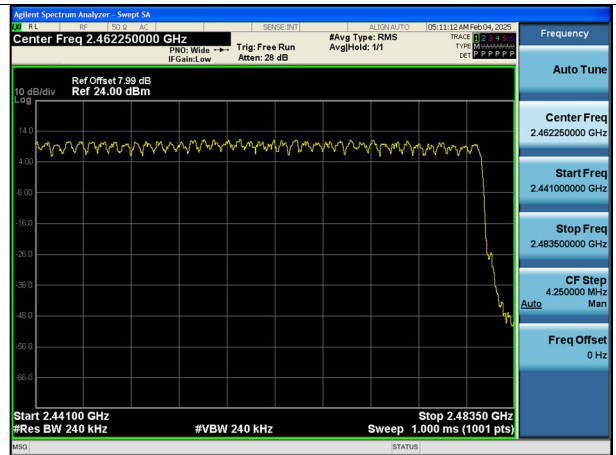
\pi/4 DQPSK (2.441 GHz - 2.483.5 GHz)
