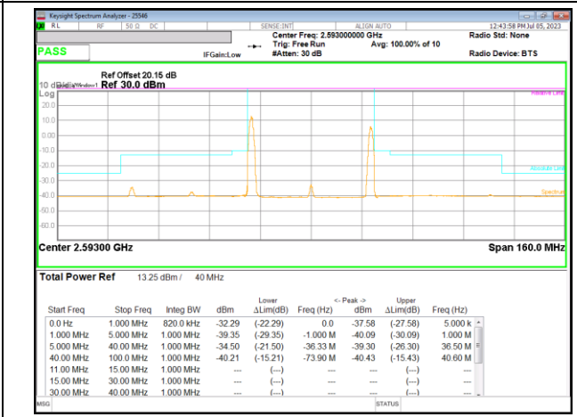
LTE B41 20MHz + 20MHz 16QAM Mid Ch RB1-0 + RB1-99
