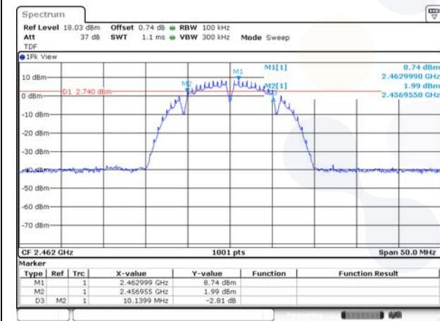
802.11b / 2 462 MHz
