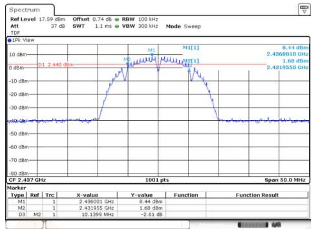
802.11b / 2 437 MHz
