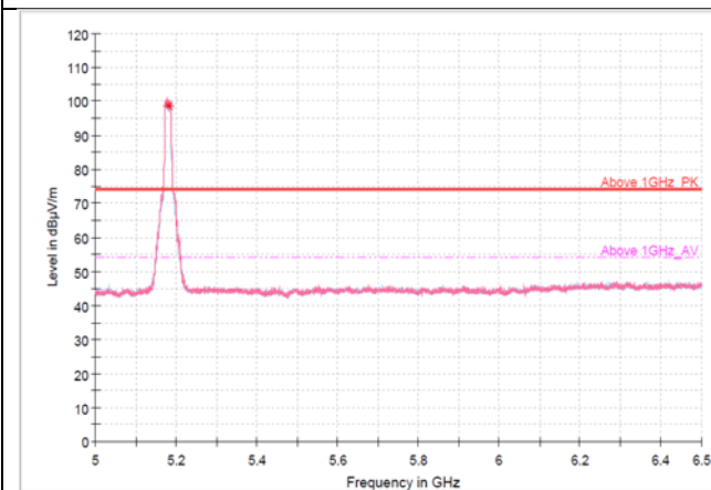
5 GHz - 6.5 GHz
