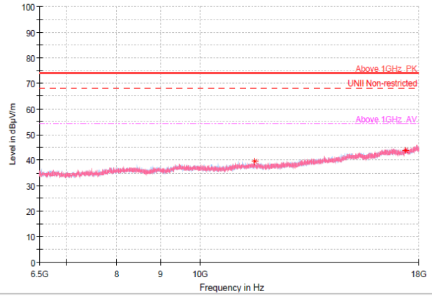
6.5 GHz - 18 GHz
