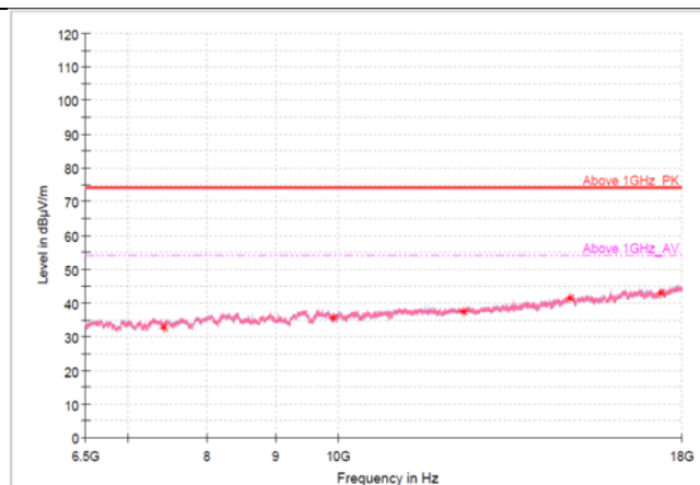
6.5 GHz - 18 GHz
