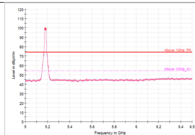
5 GHz - 6.5 GHz
