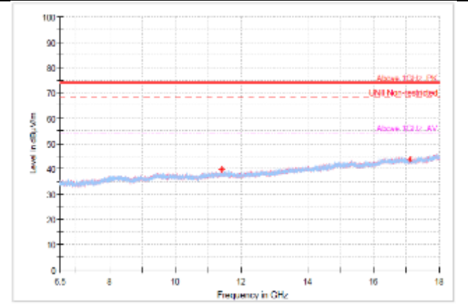
6.5 GHz - 18 GHz
