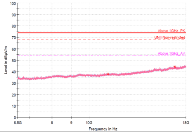
6.5 GHz - 18 GHz
