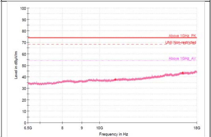
6.5 GHz - 18 GHz
