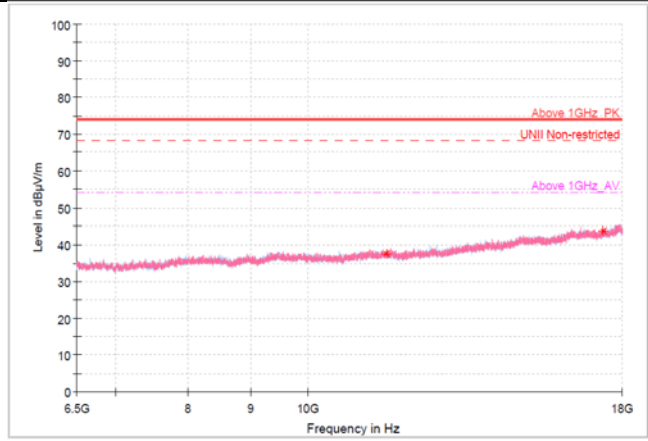
6.5 GHz - 18 GHz
