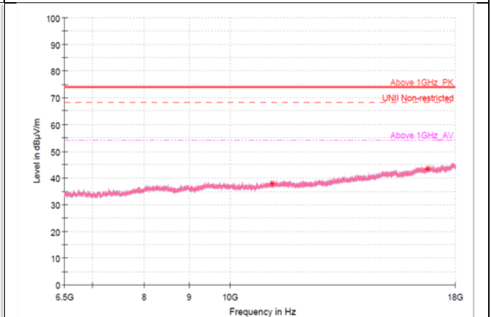
6.5 GHz - 18 GHz
