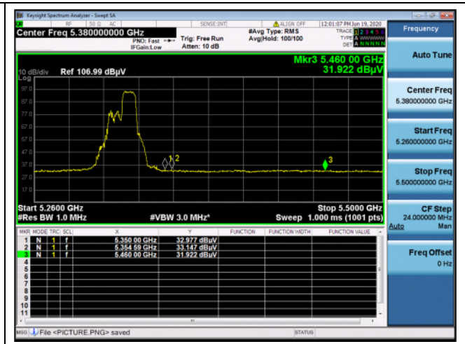
High channel_54 RU (Average)
