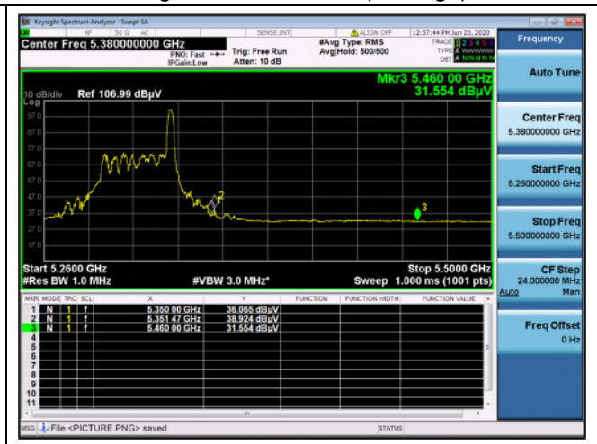
High channel_17 RU (Average)
