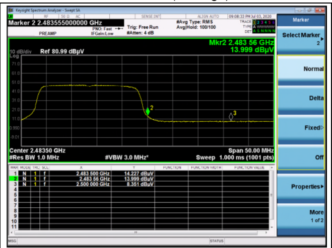
13 channel (Average)
