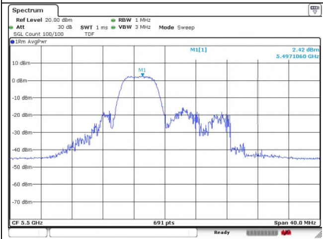
40 RU
