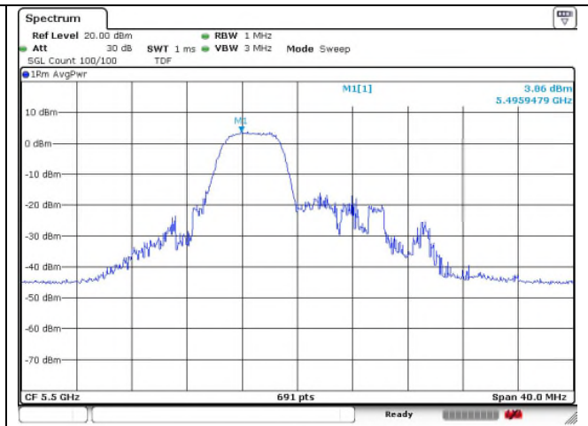
40 RU
