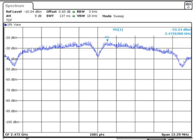
802.11b / 2 472 MHz
