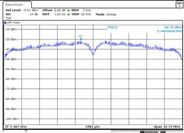
802.11b / 2 467 MHz
