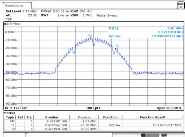
802.11b / 2 472 MHz
