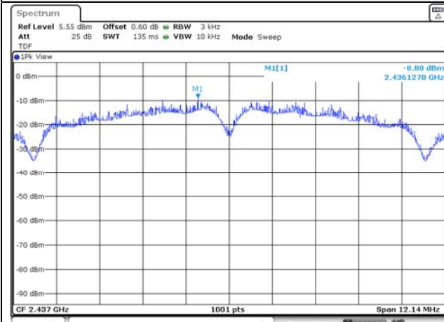
802.11b / 2 437 MHz
