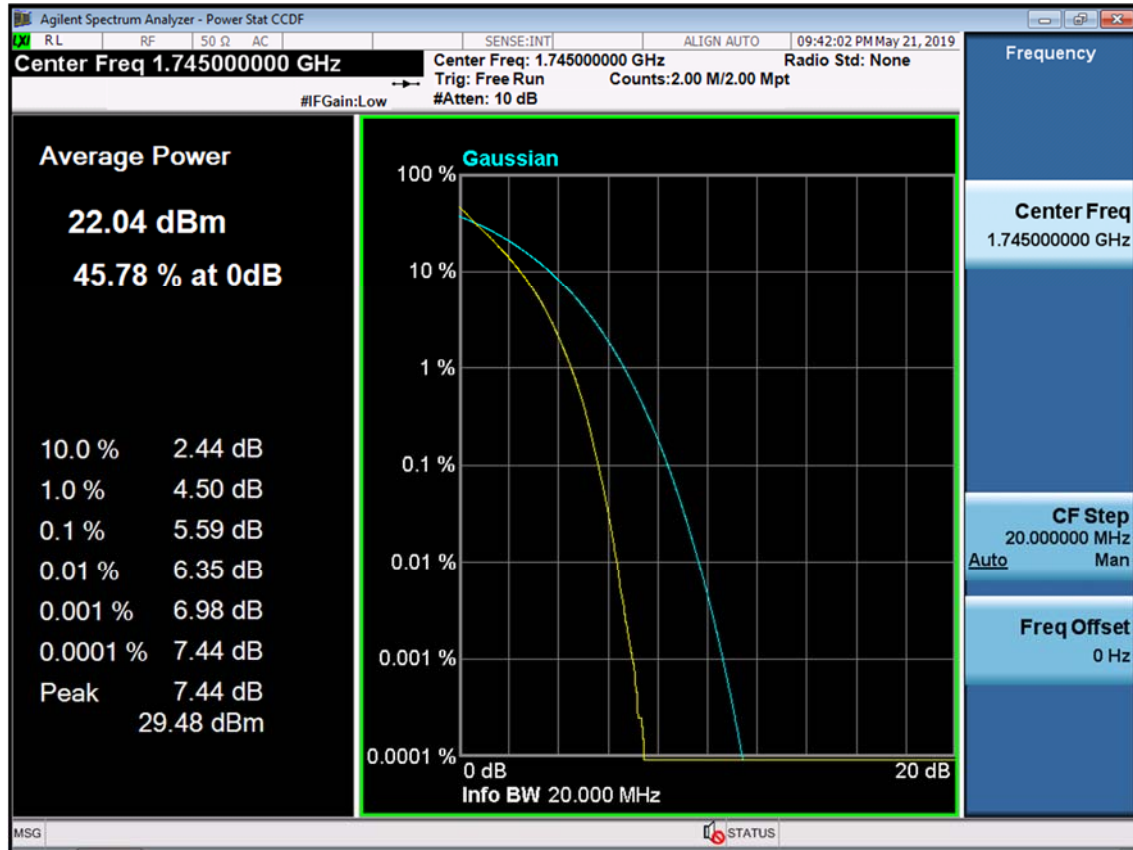
BAND 66/4. PAR Plot (20M BW_Ch.132322_QPSK_RB100_0)
