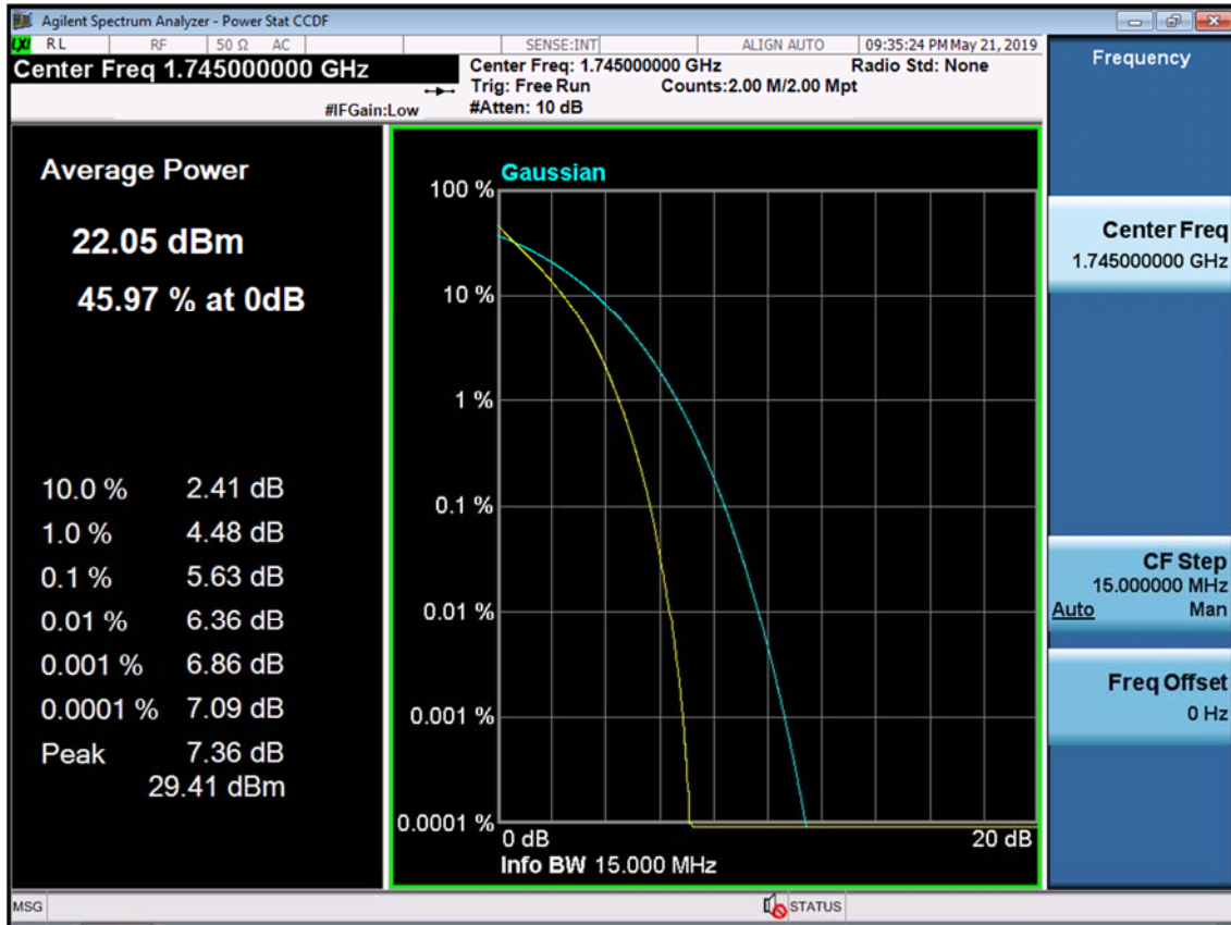
BAND 66/4. PAR Plot (15M BW_Ch.132322_QPSK_RB75_0)
