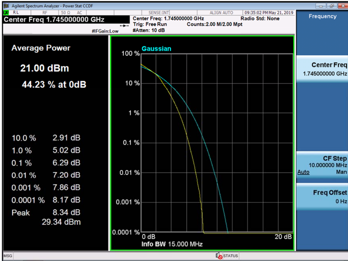
BAND 66/4. PAR Plot (15M BW_Ch.132322_16QAM_RB75_0)
