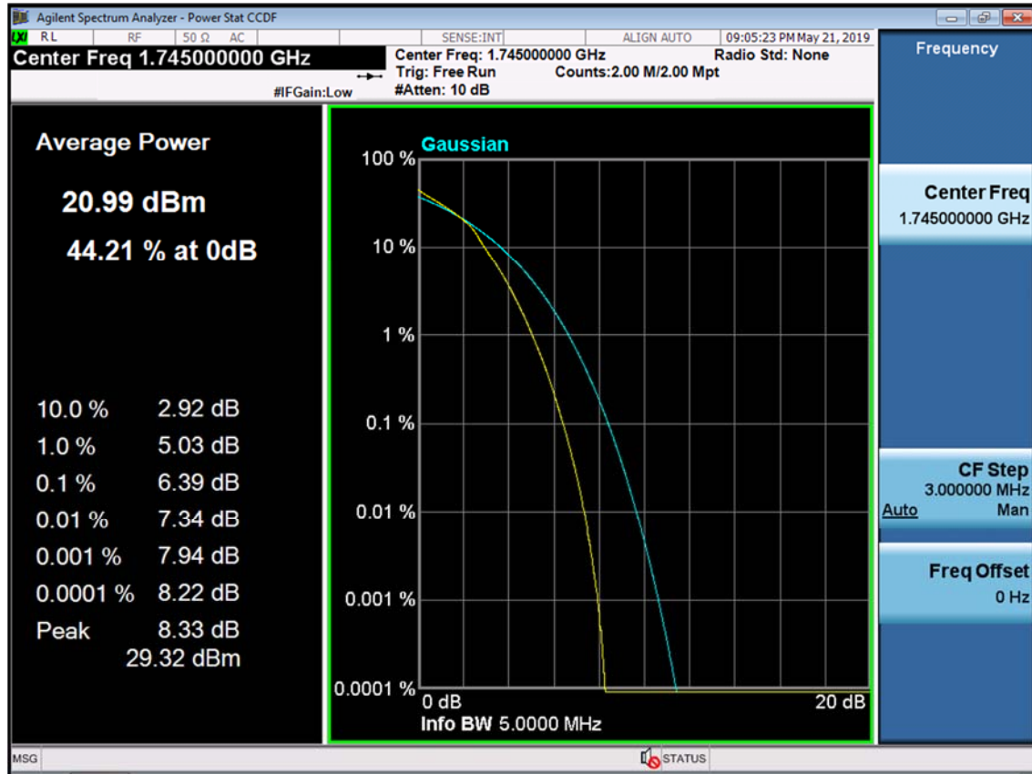
BAND 66/4. PAR Plot (5M BW_Ch.132322_16QAM_RB25_0)
