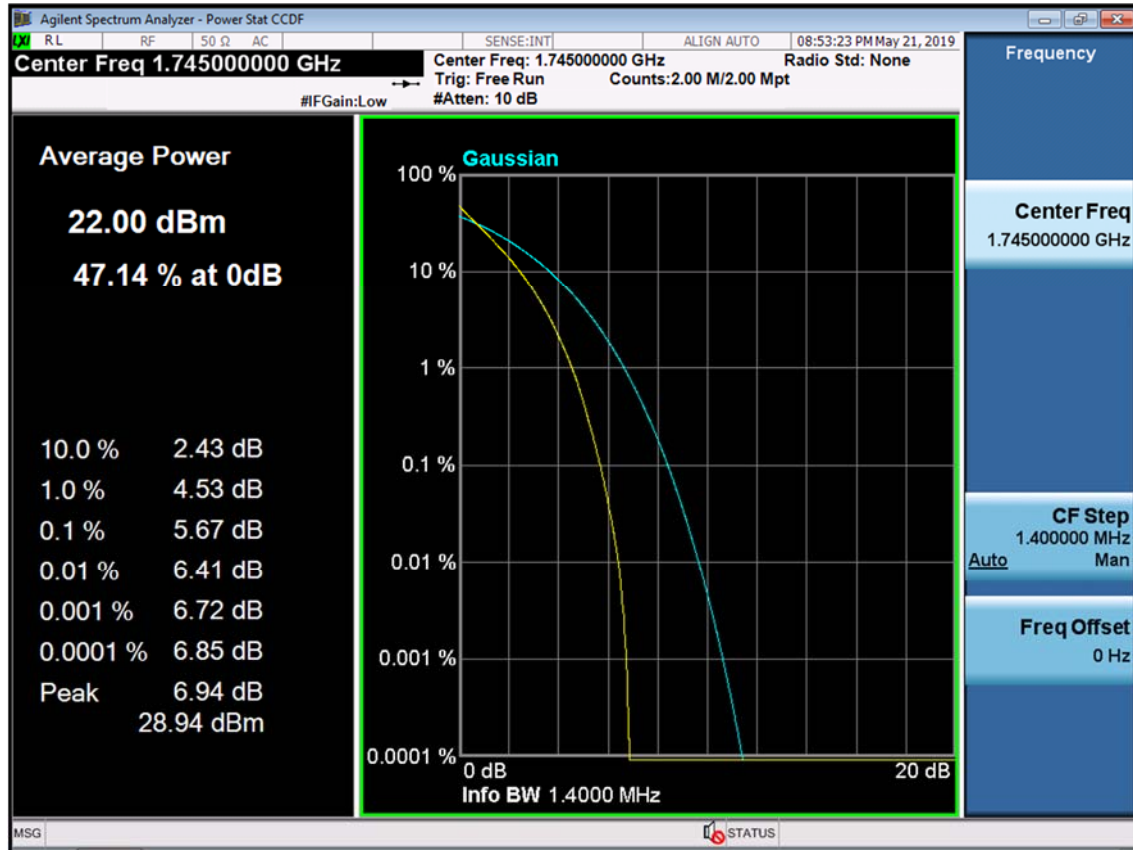
BAND 66/4. PAR Plot (1.4M BW_Ch.132322_QPSK_RB6_0)
