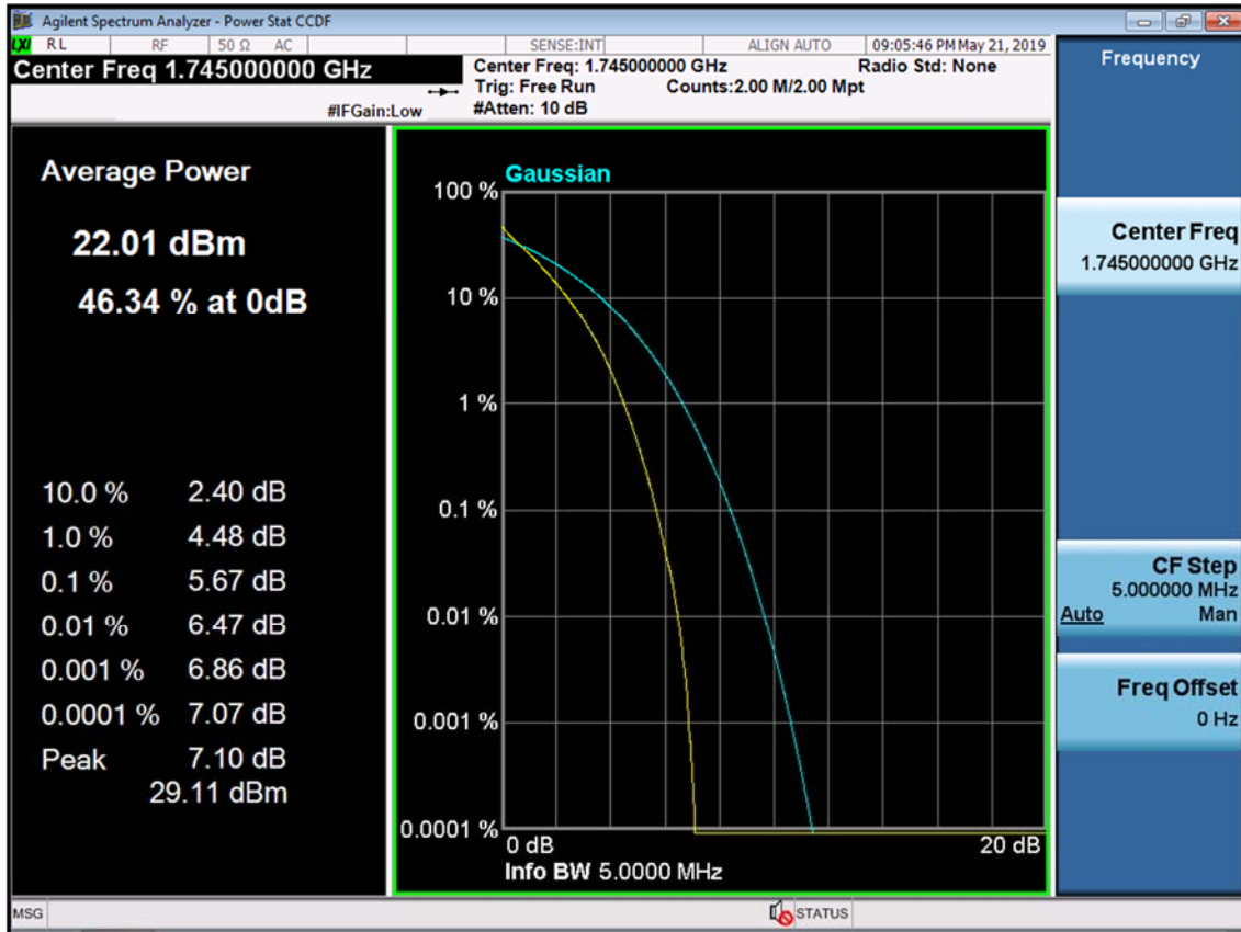
BAND 66/4. PAR Plot (5M BW_Ch.132322_QPSK_RB25_0)
