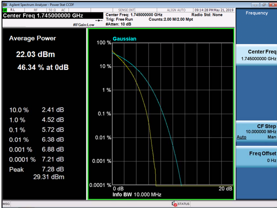
BAND 66/4. PAR Plot (10M BW_Ch.132322_QPSK_RB50_0)
