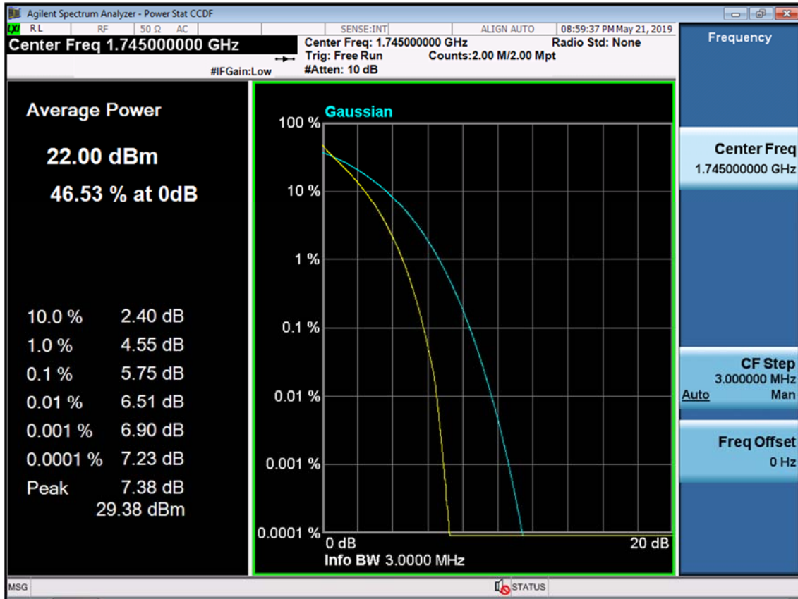
BAND 66/4. PAR Plot (3M BW_Ch.132322_QPSK_RB15_0)
