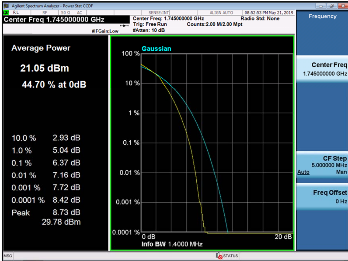
BAND 66/4. PAR Plot (1.4M BW_Ch.132322_16QAM_RB6_0)
