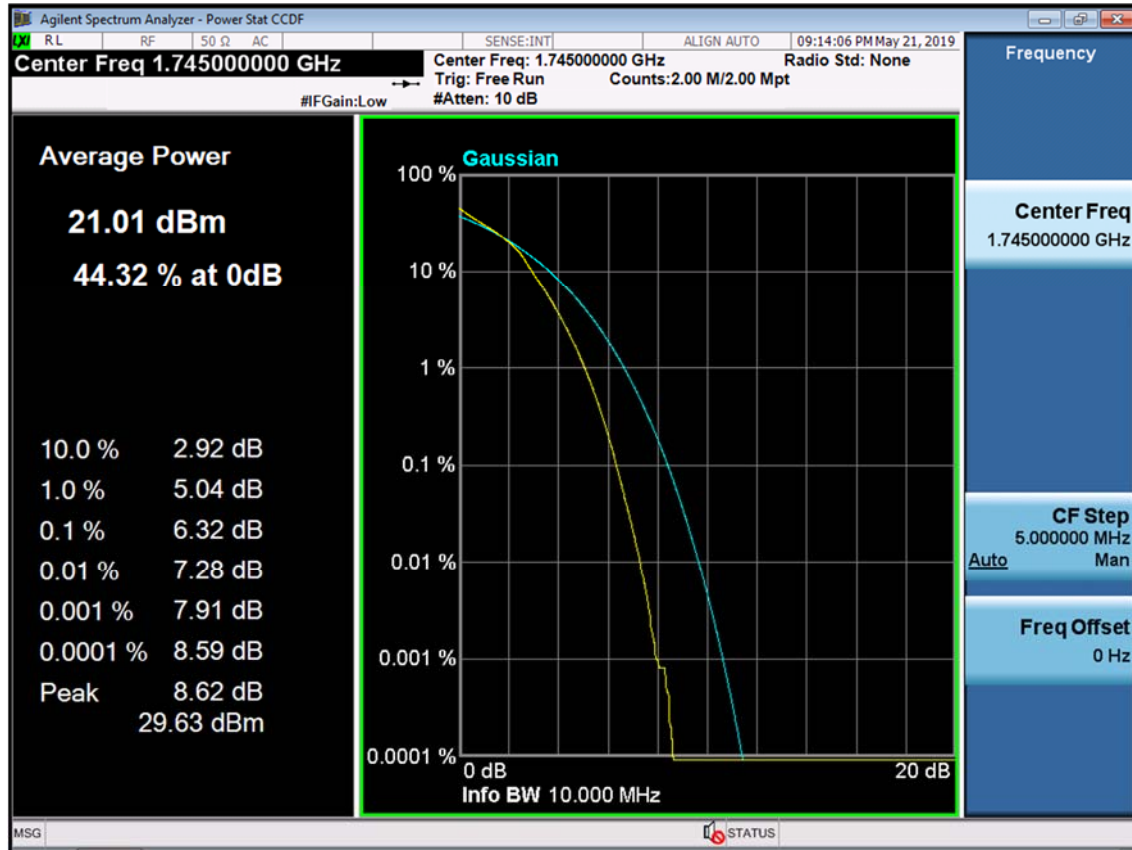
BAND 66/4. PAR Plot (10M BW_Ch.132322_16QAM_RB50_0)
