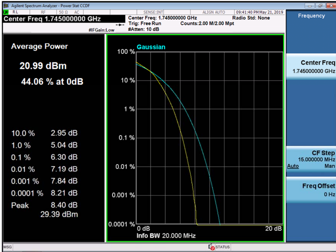
BAND 66/4. PAR Plot (20M BW_Ch.132322_16QAM_RB100_0)
