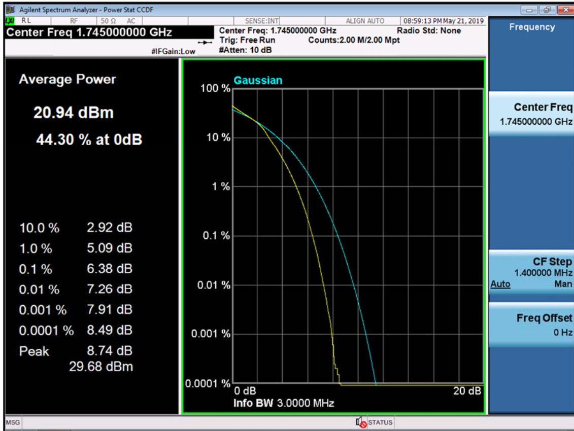
BAND 66/4. PAR Plot (3M BW_Ch.132322_16QAM_RB15_0)
