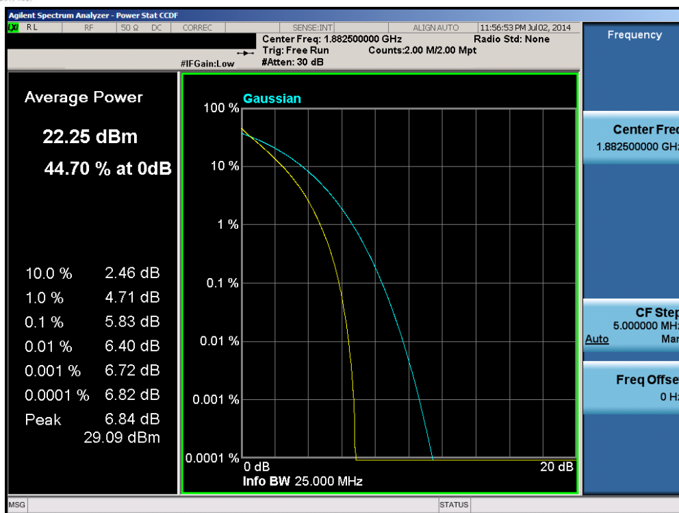
Plot 6-27. PAR Plot (Band 25 – 15.0MHz QPSK – RB Size 75)
