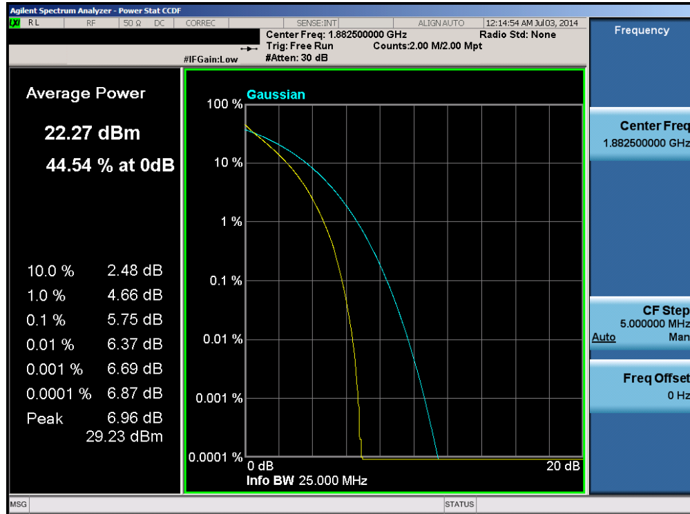
Plot 6-29. PAR Plot (Band 25 – 20.0MHz QPSK – RB Size 100)
