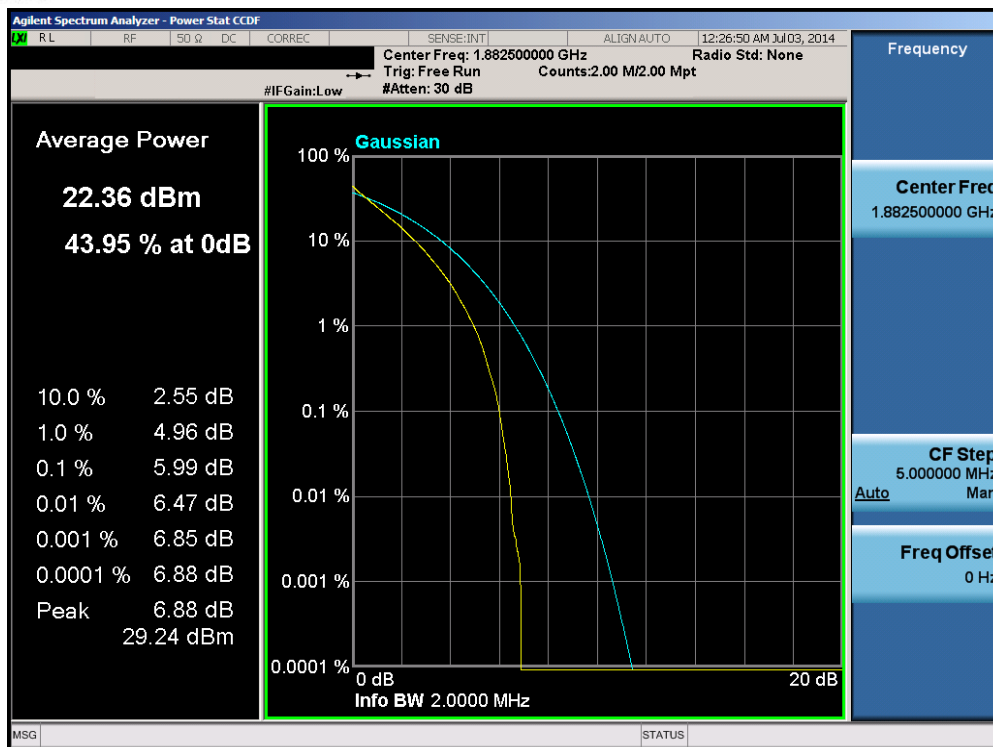
Plot 6-25. PAR Plot (Band 25 – 1.4MHz QPSK – RB Size 6)
