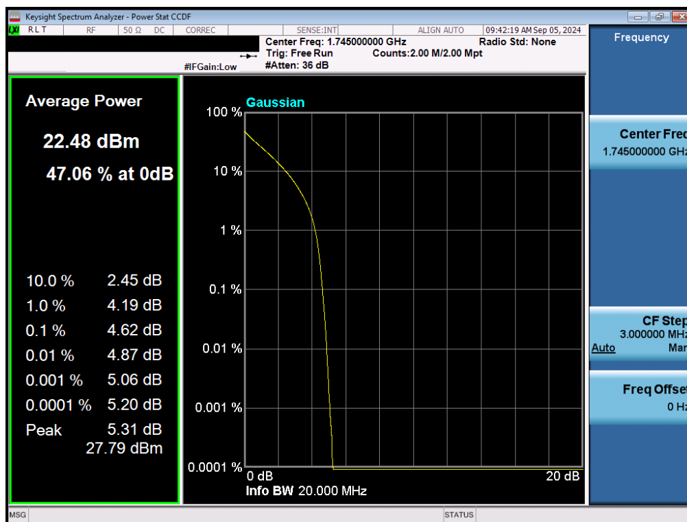
Plot 7-168. PAR Plot (LTE Band 66/4 - 20MHz QPSK - Full RB - ANT1)
