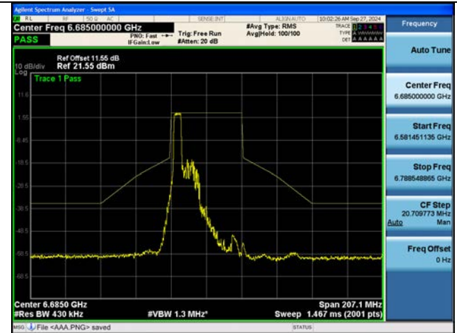
802.11be EHT40M Ch.147(6685 MHz) 242 Tones 61 RU
