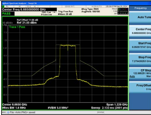
802.11be EHT160M Ch.143(6665 MHz) SU
