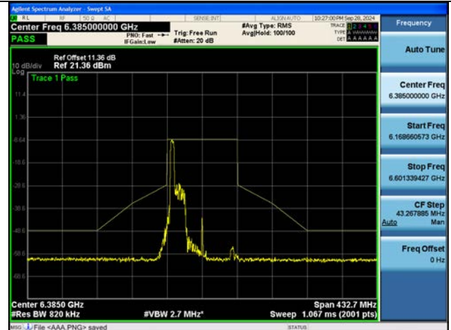
802.11be EHT80M Ch.87(6385 MHz) 242 Tones 61 RU
