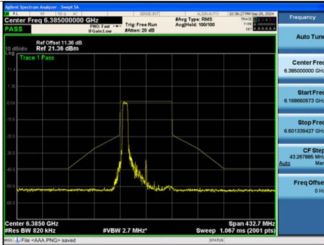
802.11be EHT80M Ch.87(6385 MHz) 484 Tones 65 RU
