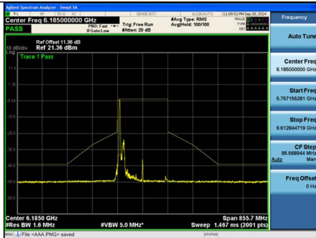
802.11be EHT160M Ch.47(6185 MHz) 106 Tones 53 RU
