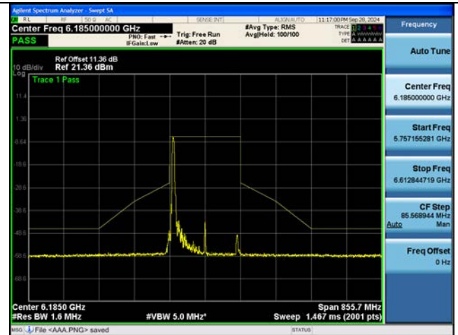
802.11be EHT160M Ch.47(6185 MHz) 242 Tones 61 RU
