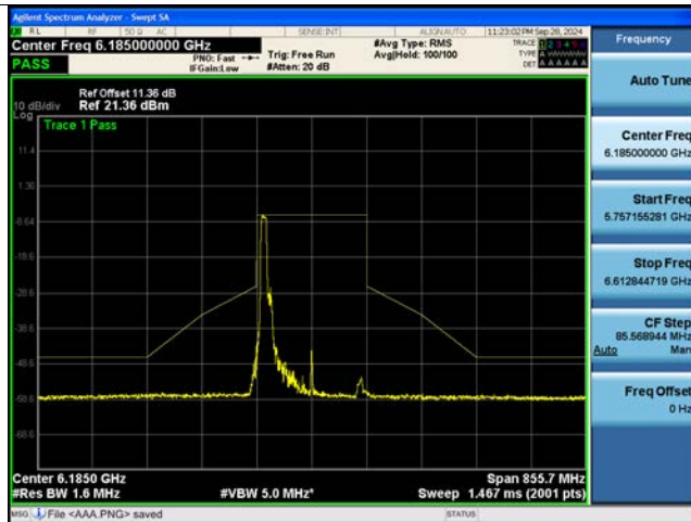
802.11be EHT160M Ch.47(6185 MHz) 484 Tones 65 RU
