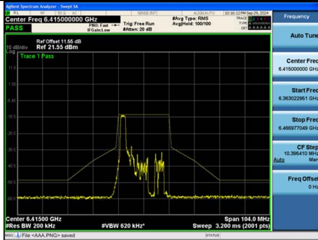
802.11be EHT20M Ch.93(6415 MHz) 106 Tones 53 RU
