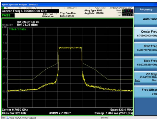
802.11be EHT80M Ch.151(6705 MHz) 996 Tones 67 RU
