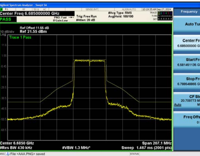
802.11be EHT40M Ch.147(6685 MHz) 484 Tones 65 RU
