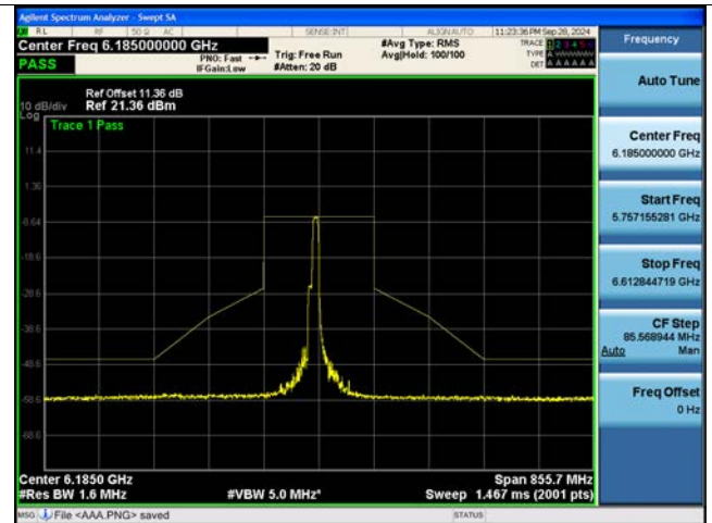
802.11be EHT160M Ch.47(6185 MHz) 996 Tones 67 RU
