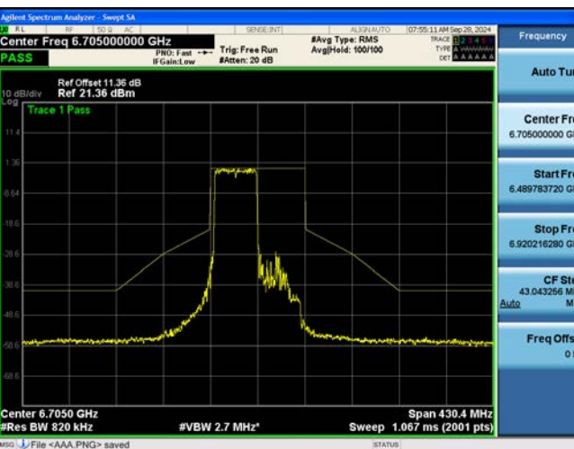
802.11be EHT80M Ch.151(6705 MHz) 484 Tones 65 RU
