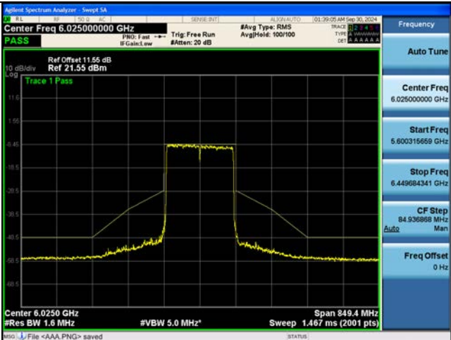
802.11be EHT160M Ch.15(6025 MHz) 2x996 Tones 68 RU
