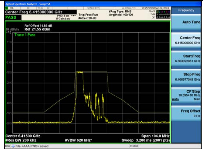
802.11be EHT20M Ch.93(6415 MHz) 242 Tones 61 RU
