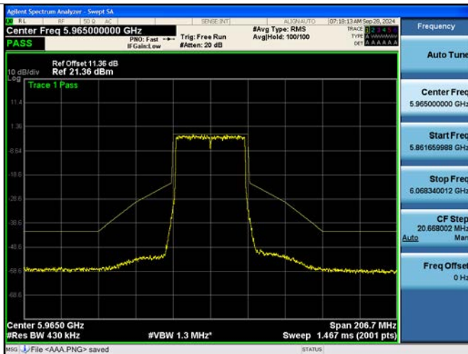
802.11be EHT40M Ch.3(5965 MHz) SU
