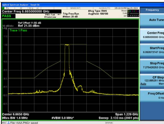
802.11be EHT160M Ch.143(6665 MHz) 484 Tones 65 RU
