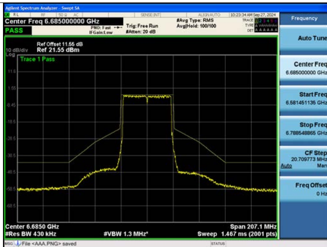
802.11be EHT40M Ch.147(6685 MHz) SU
