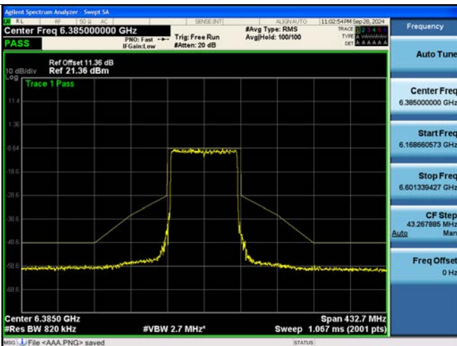
802.11be EHT80M Ch.87(6385 MHz) 996 Tones 67 RU
