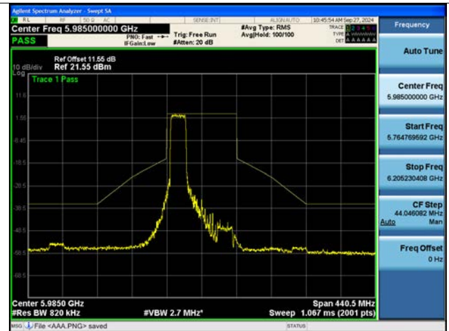
802.11be EHT80M Ch.7(5985 MHz) 996 Tones 67 RU
