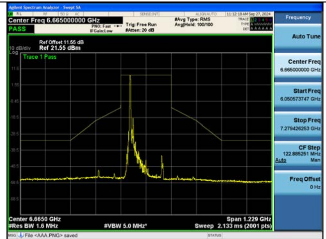
802.11be EHT160M Ch.143(6665 MHz) 242 Tones 61 RU
