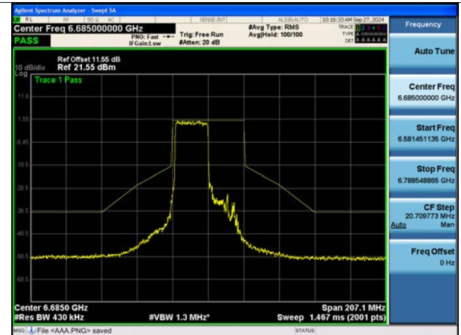
802.11be EHT40M Ch.147(6685 MHz) SU
