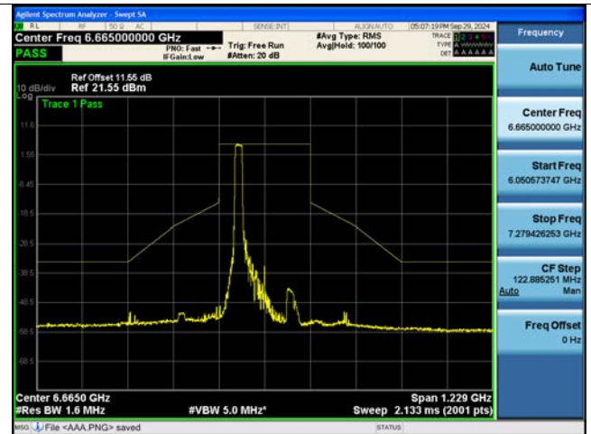
802.11be EHT160M Ch.143(6665 MHz) 996 Tones 67 RU
