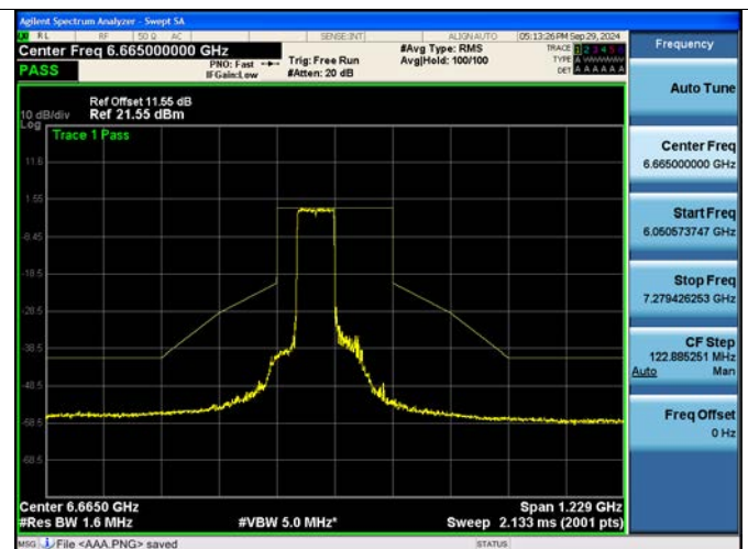
802.11be EHT160M Ch.143(6665 MHz) 996 Tones 67 RU
