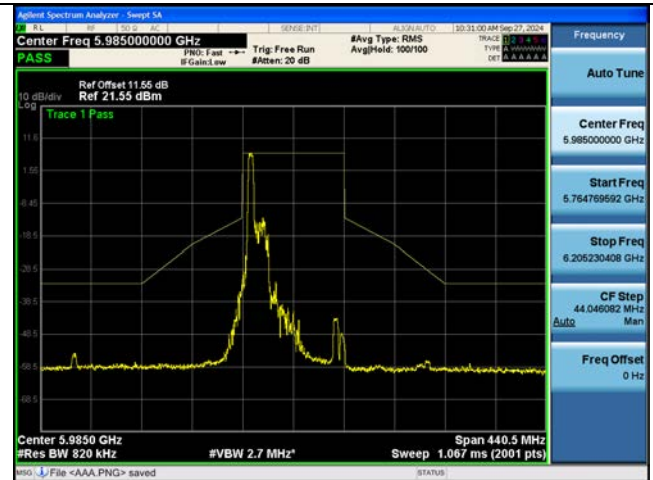
802.11be EHT80M Ch.7(5985 MHz) 242 Tones 61 RU
