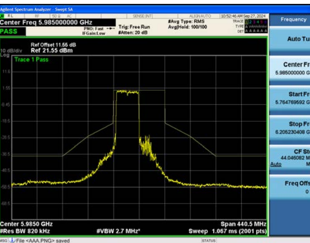
802.11be EHT80M Ch.7(5985 MHz) 484 Tones 65 RU
