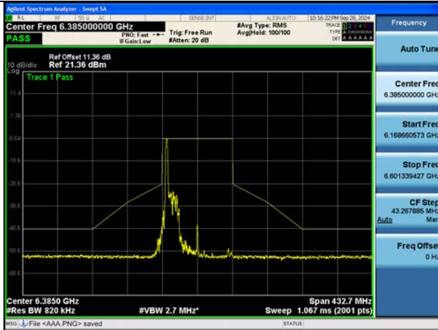
802.11be EHT80M Ch.87(6385 MHz) 106 Tones 53 RU
