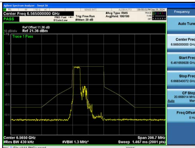
802.11be EHT40M Ch.123(6565 MHz) 484 Tones 65 RU
