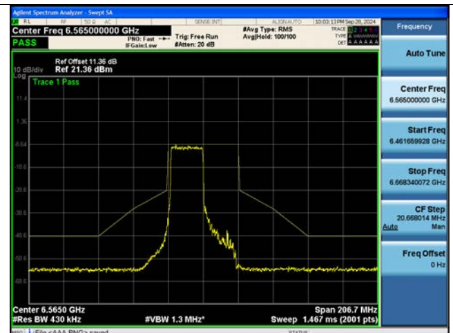
802.11be EHT40M Ch.123(6565 MHz) SU
