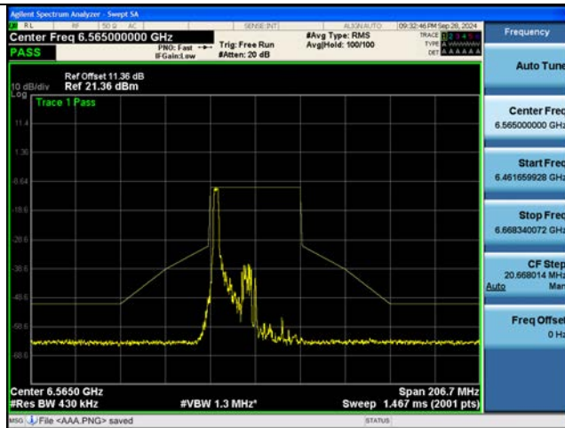
802.11be EHT40M Ch.123(6565 MHz) 106 Tones 53 RU
