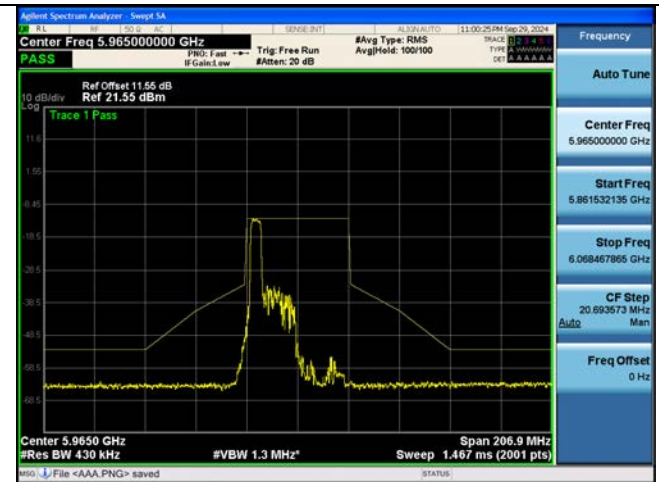
802.11be EHT40M Ch.3(5965 MHz) 242 Tones 61 RU
