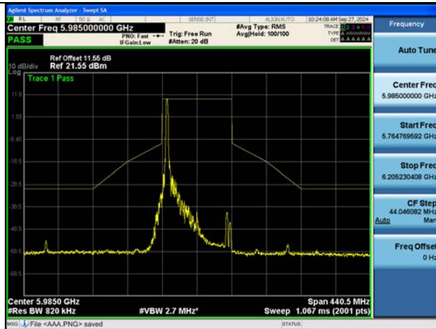
802.11be EHT80M Ch.7(5985 MHz) 106 Tones 53 RU
