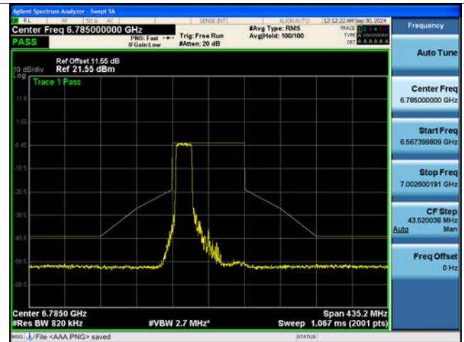
802.11be EHT80M Ch.167(6785 MHz) 996 Tones 67 RU
