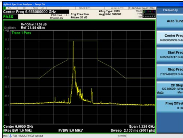
802.11be EHT160M Ch.143(6665 MHz) 106 Tones 53 RU
