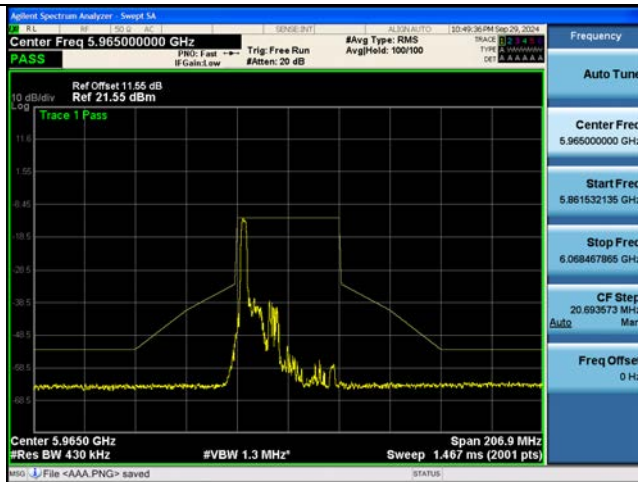
802.11be EHT40M Ch.3(5965 MHz) 106 Tones 53 RU
