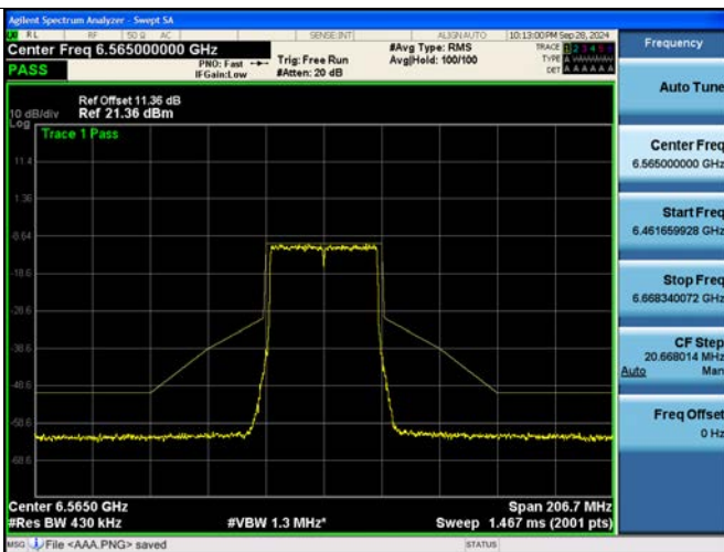
802.11be EHT40M Ch.123(6565 MHz) SU
