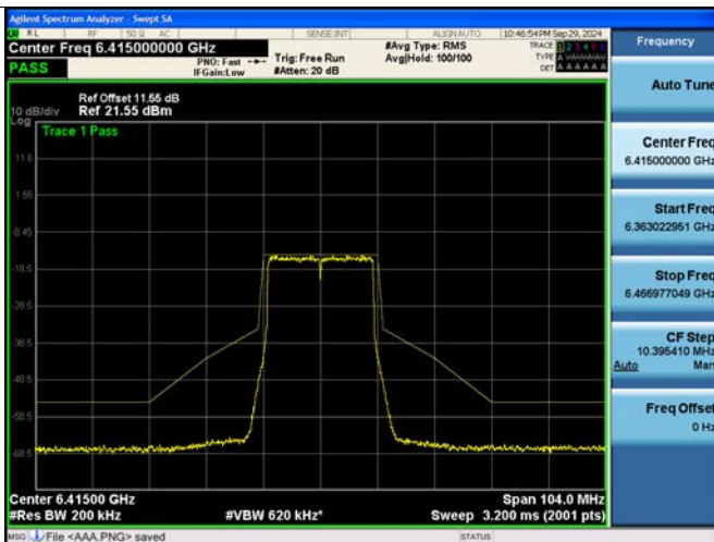
802.11be EHT20M Ch.93(6415 MHz) SU
