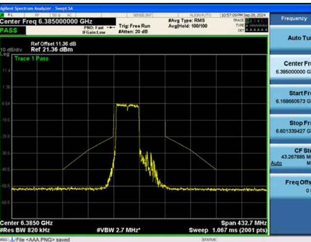
802.11be EHT80M Ch.87(6385 MHz) 484 Tones 65 RU
