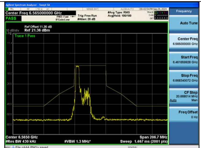
802.11be EHT40M Ch.123(6565 MHz) 242 Tones 61 RU
