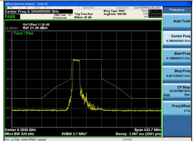
802.11be EHT80M Ch.87(6385 MHz) 996 Tones 67 RU
