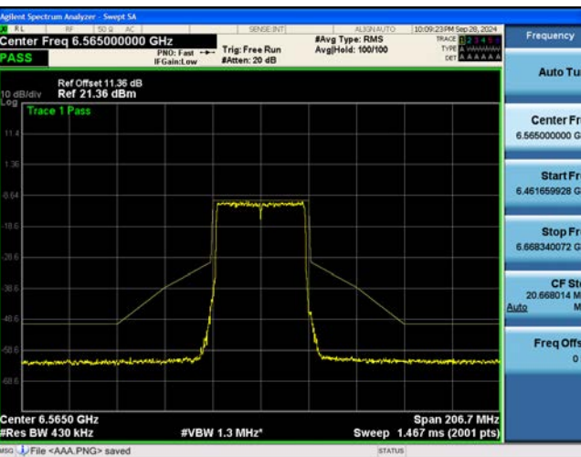
802.11be EHT40M Ch.123(6565 MHz) 484 Tones 65 RU
