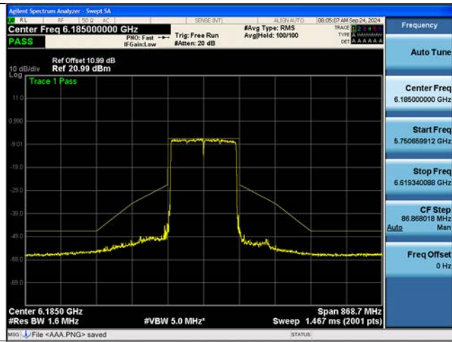
802.11be EHT160M Ch.47(6185 MHz) 2x996 Tones 68 RU
