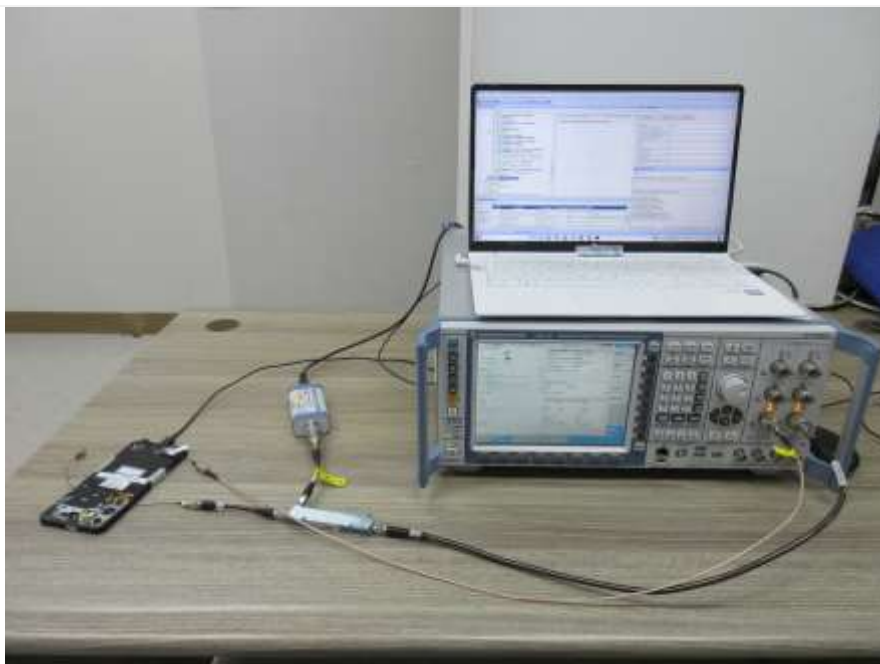
Test setup photo-6 (8-1(d) WLAN)
