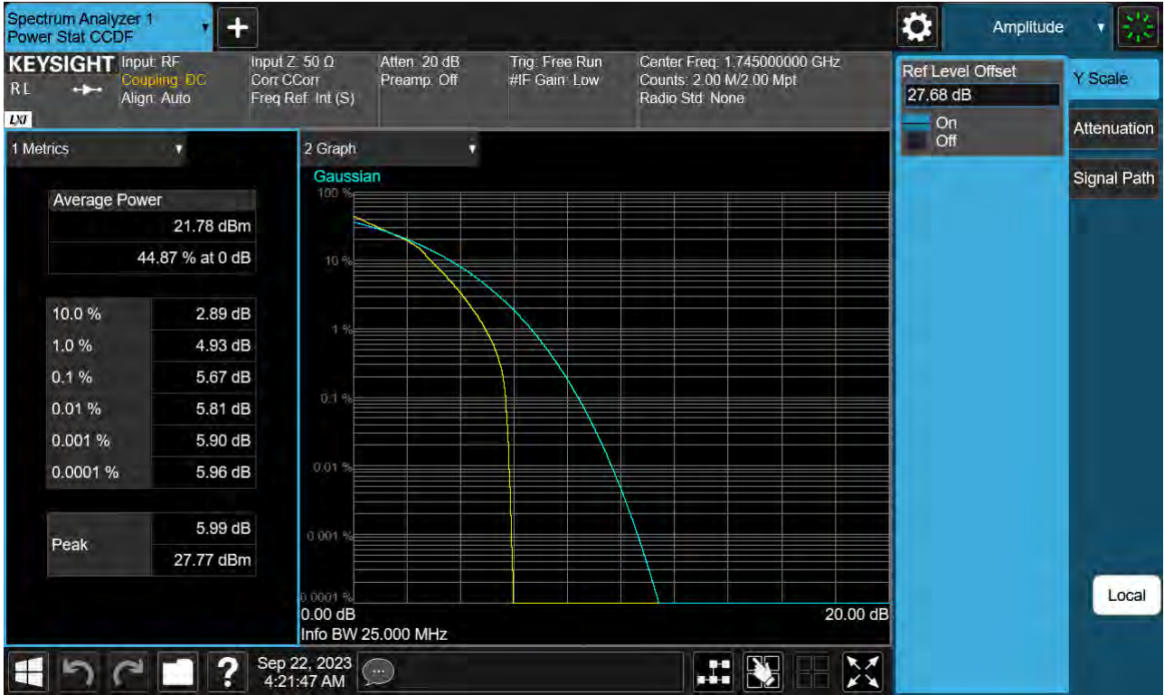
Sub6 n66. PAR Plot (25 M BW_Ch.349000_16QAM_Full RB)
