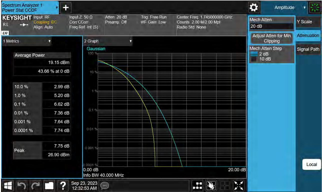
Sub6 n66. PAR Plot (40 M BW_Ch.349000_256QAM_Full RB)
