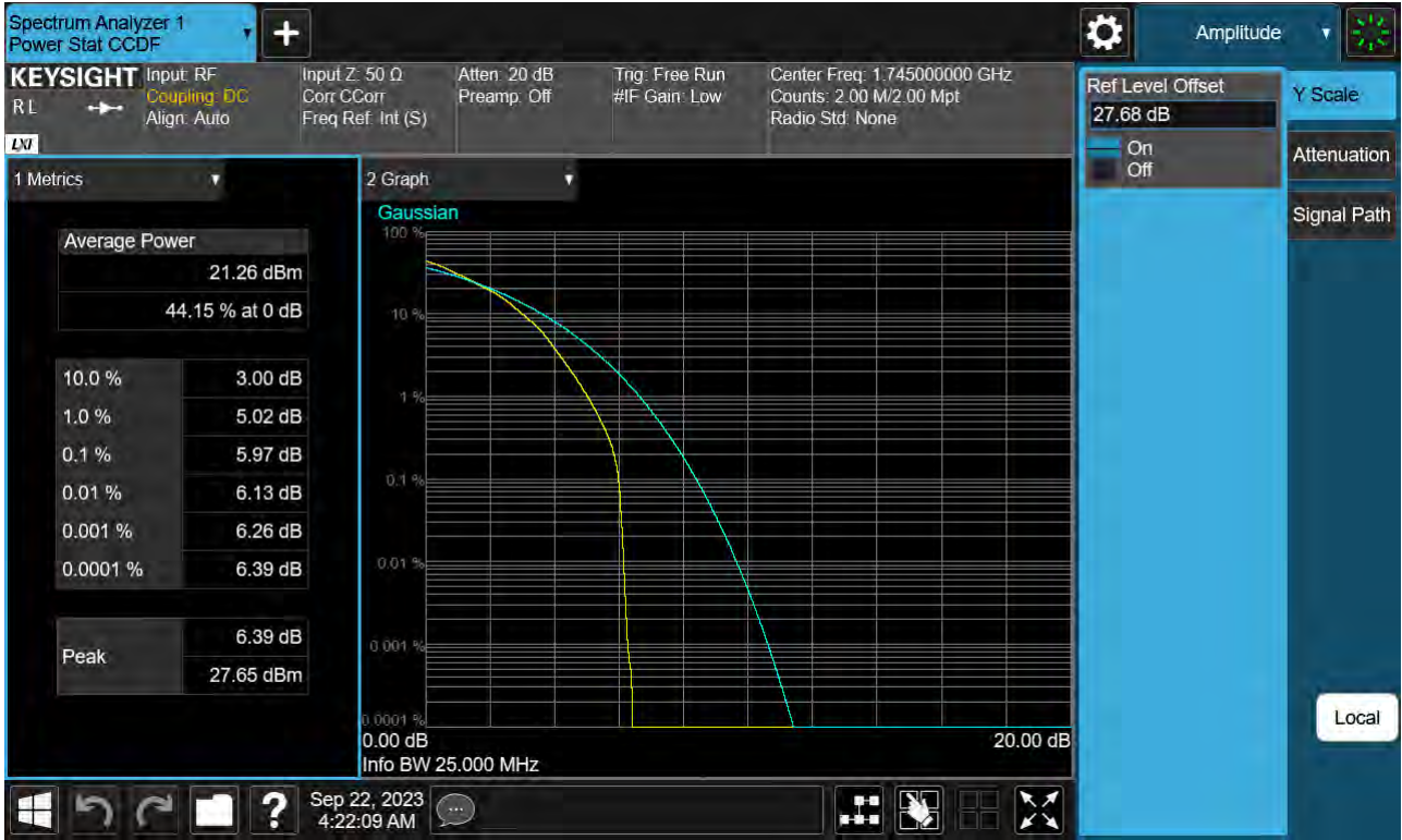
Sub6 n66. PAR Plot (25 M BW_Ch.349000_64QAM_Full RB)
