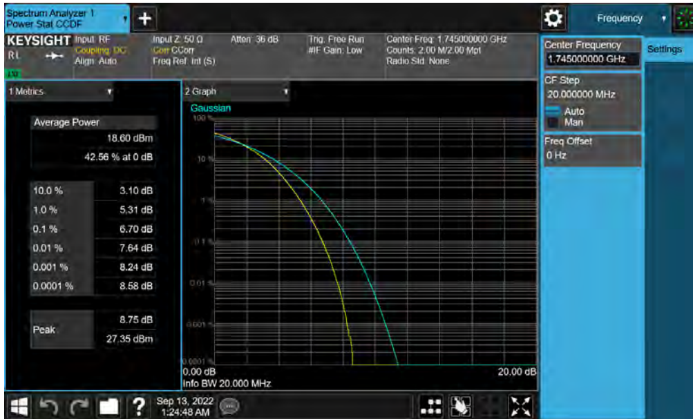
Plot 7-99. PAR Plot (LTE Band 66/4 - 20MHz 256-QAM - Full RB)
