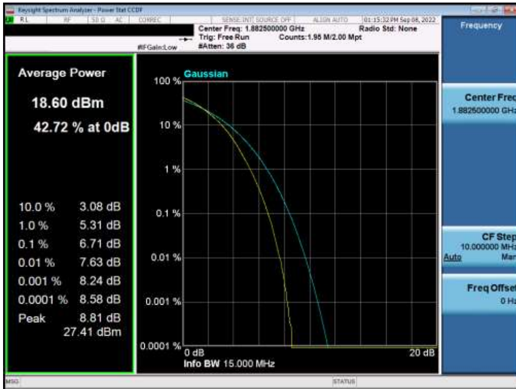
Plot 7-62. PAR Plot (LTE Band 2 - 15MHz 256-QAM - Full RB)
