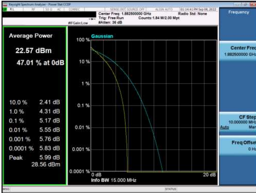
Plot 7-61. PAR Plot (LTE Band 2 - 15MHz QPSK - Full RB)
