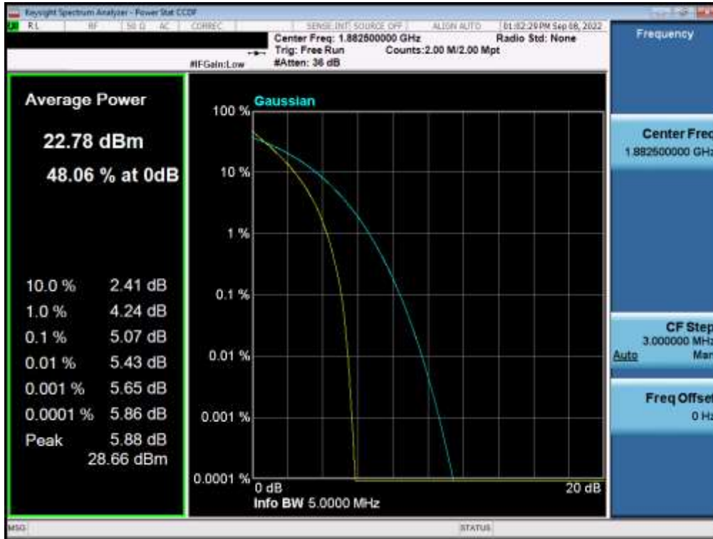
Plot 7-65. PAR Plot (LTE Band 2 - 5MHz QPSK - Full RB)
