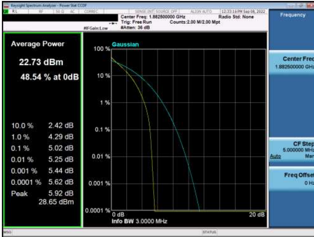
Plot 7-67. PAR Plot (LTE Band 2 - 3MHz QPSK - Full RB)
