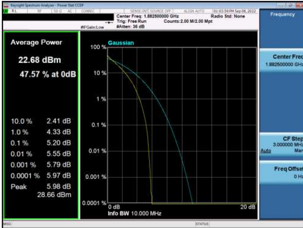
Plot 7-63. PAR Plot (LTE Band 2 - 10MHz QPSK - Full RB)
