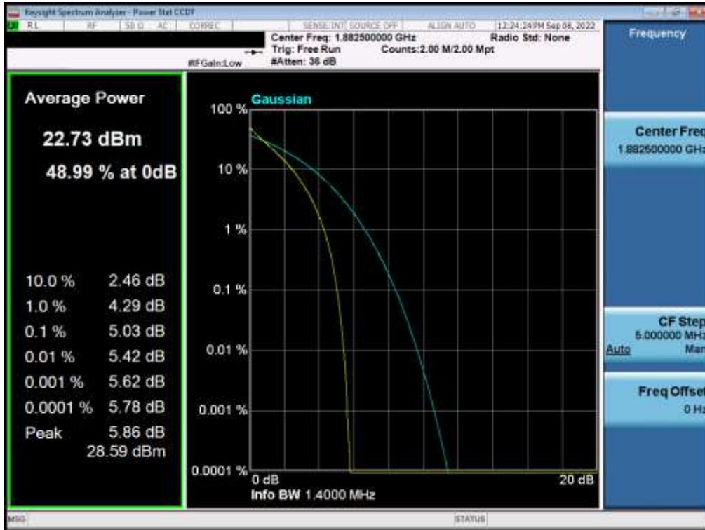
Plot 7-69. PAR Plot (LTE Band 2 - 1.4MHz QPSK - Full RB)
