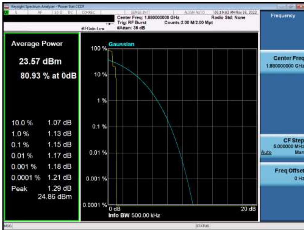
Plot 7-72. PAR Plot (EDGE, Ch. 661)
