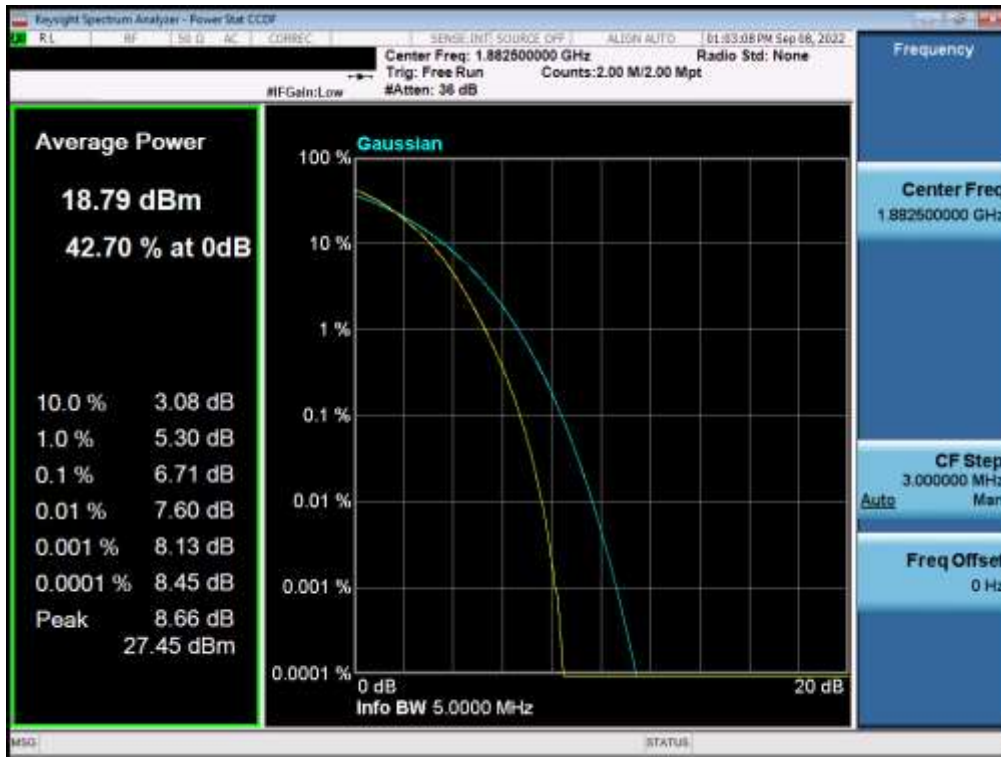
Plot 7-66. PAR Plot (LTE Band 2 - 5MHz 256-QAM - Full RB)
