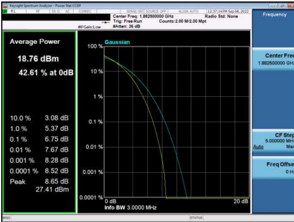
Plot 7-68. PAR Plot (LTE Band 2 - 3MHz 256-QAM - Full RB)
