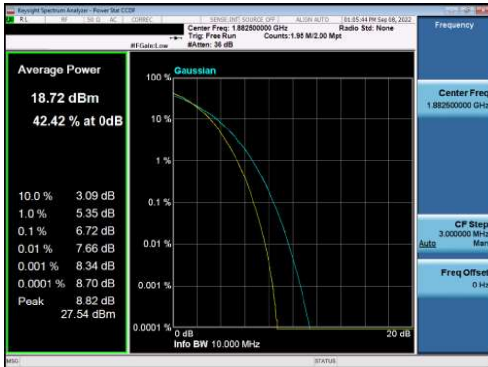
Plot 7-64. PAR Plot (LTE Band 2 - 10MHz 256-QAM - Full RB)
