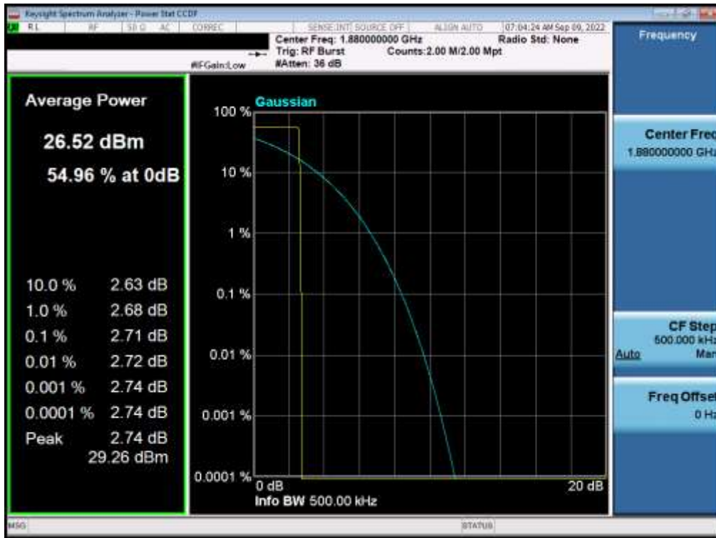
Plot 7-71. PAR Plot (GPRS, Ch. 661)
