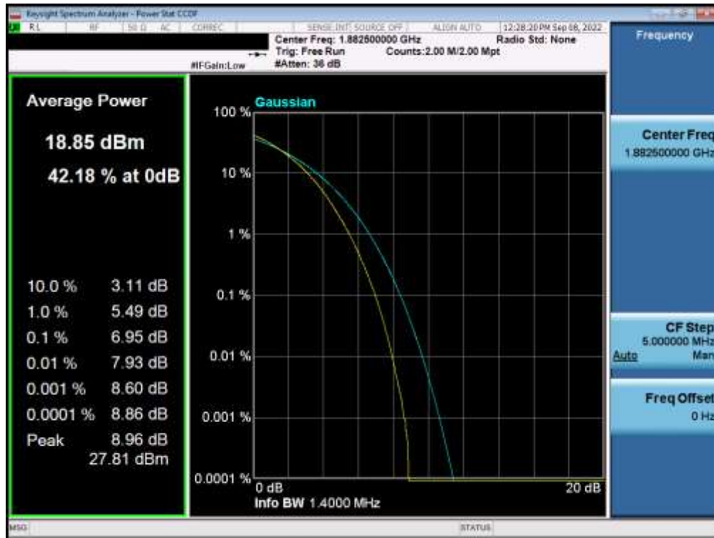
Plot 7-70. PAR Plot (LTE Band 2 - 1.4MHz 256-QAM - Full RB)
