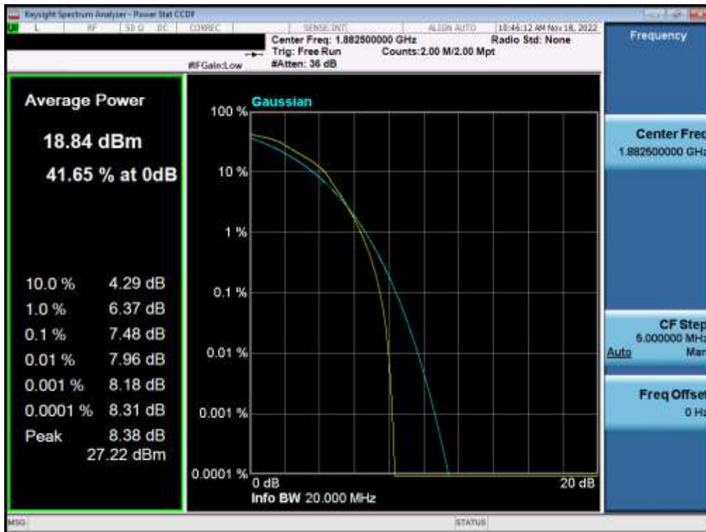
Plot 7-60. PAR Plot (LTE Band 2 - 20MHz 256-QAM - Full RB)
