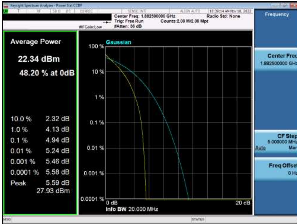
Plot 7-59. PAR Plot (LTE Band 2 - 20MHz QPSK - Full RB)
