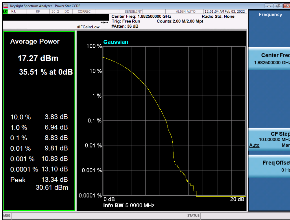
Plot 7-57. PAR Plot (NR Band n25/2 - 5.0MHz CP-OFDM 256-QAM - Full RB)
