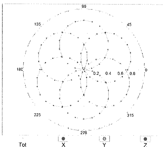
f=1800 MHz,R22
