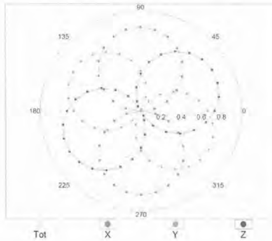
f=1800 MHz,R22
