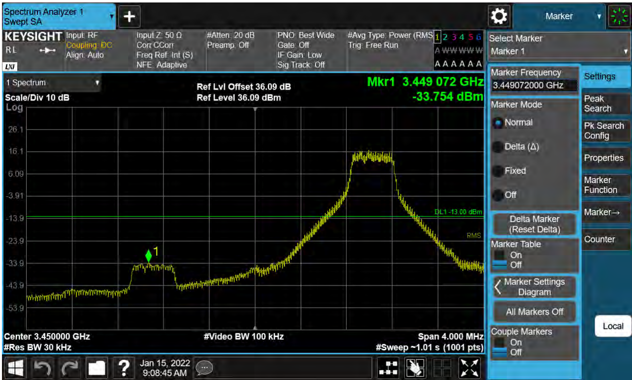
Sub6 n77. Low Band Edge Plot (100 M BW Ch.633334 BPSK 1RB)(1)
