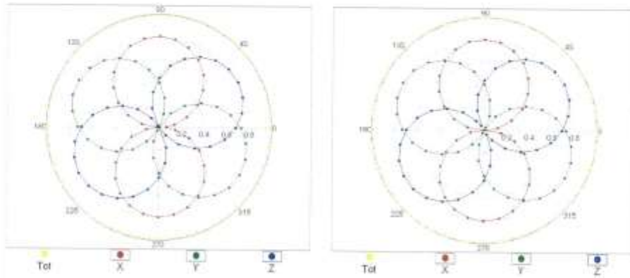
f=1800 MHz,R22
