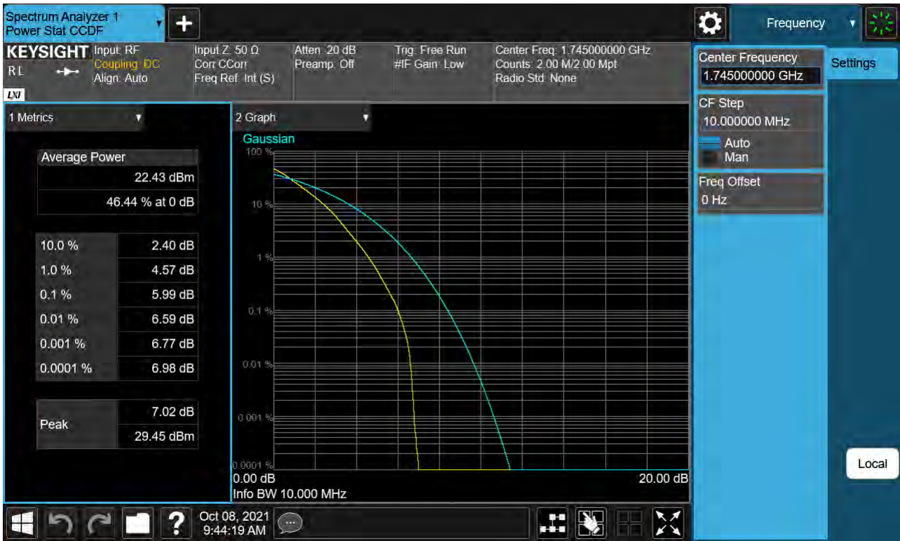
Sub6 n66. PAR Plot (10 M BW_Ch.349000_QPSK_Full RB)
