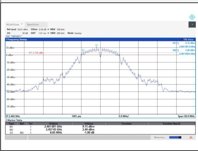
802.11b / 2 462 MHz
