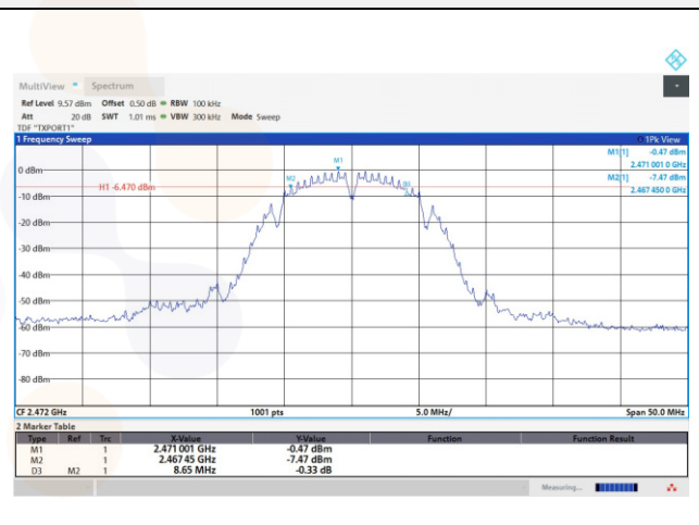
802.11b / 2 472 MHz
