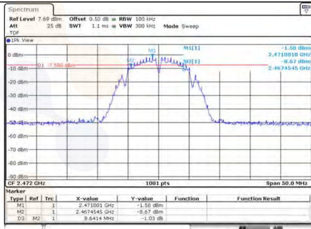
802.11b / 2 472 MHz
