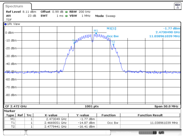
802.11b / 2 472 MHz
