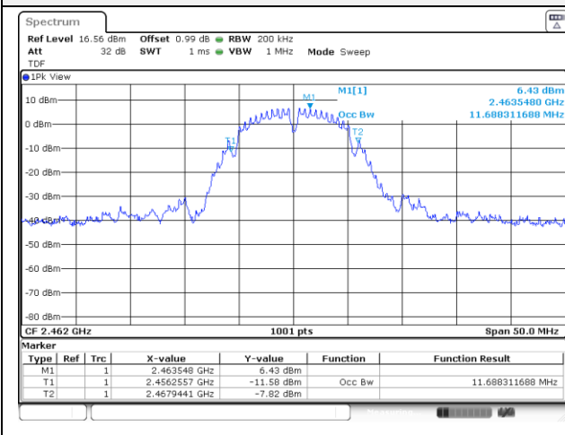
802.11b / 2 462 MHz
