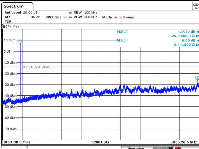
EDR(8DPSK)_2 441 MHz
