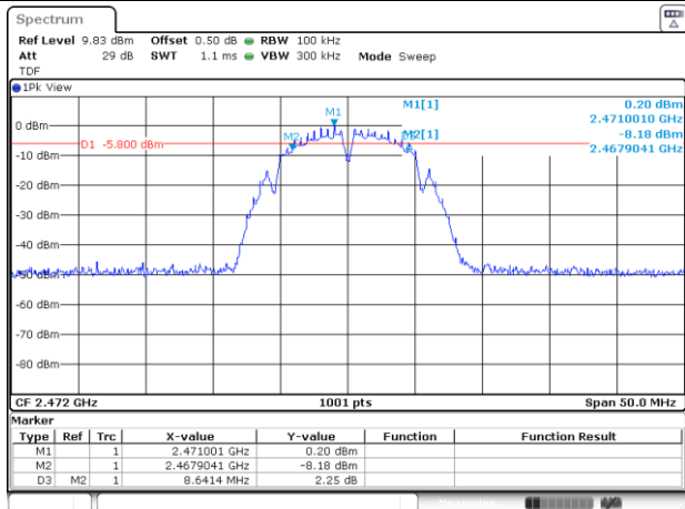
802.11b / 2 472 MHz
