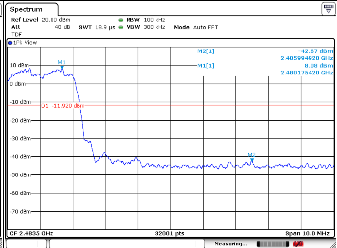
EDR(8DPSK)_Hopping_High edge
