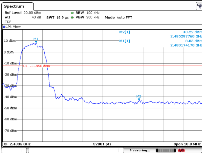
EDR(8DPSK)_2 480 MHz
