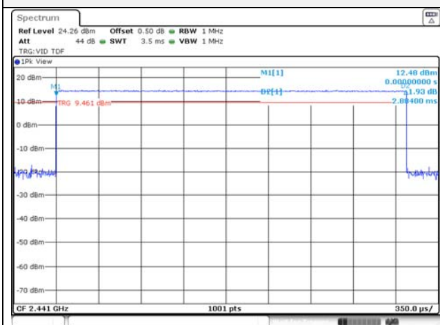
GFSK / DH5
