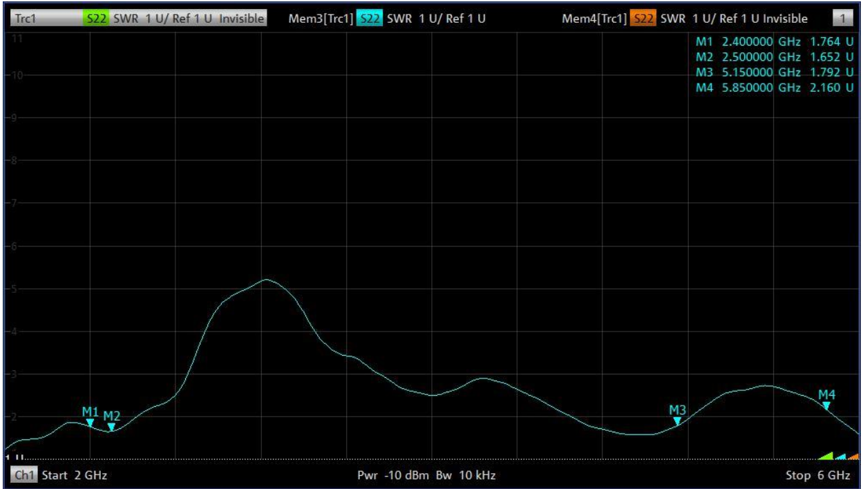
BT/WiFi Antenna
