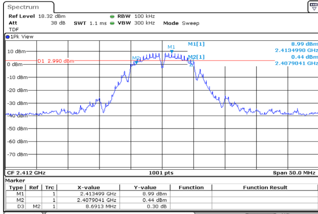
802.11b / 2 412 MHz
