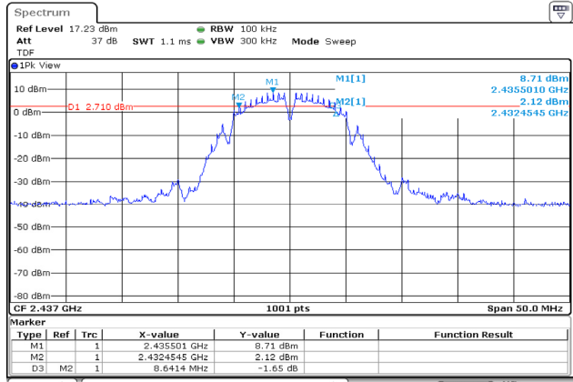
802.11b / 2 437 MHz
