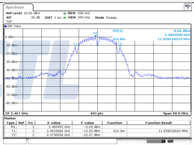
802.11b / 2 467 MHz
