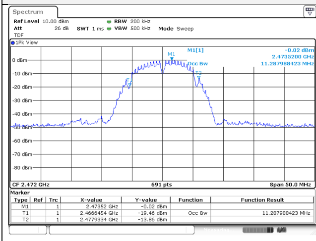
802.11b / 2 472 MHz
