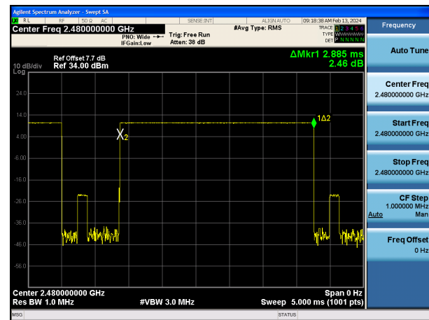
GFSK : (Ch. 78)
