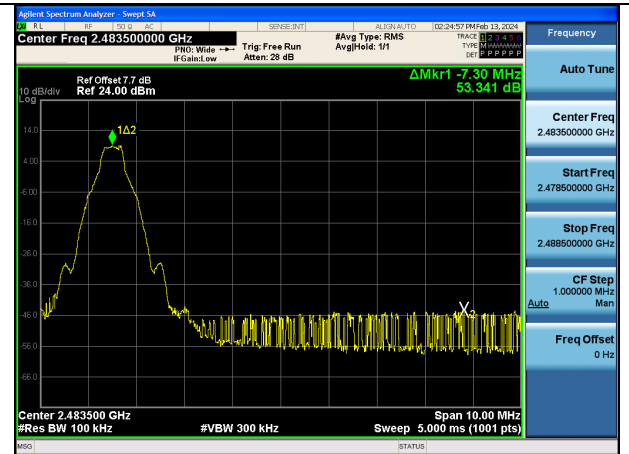
8DPSK Upper Band Edge(Ch. 78)
