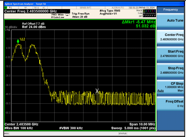
8DPSK Upper Band Edge(Ch. 78)
