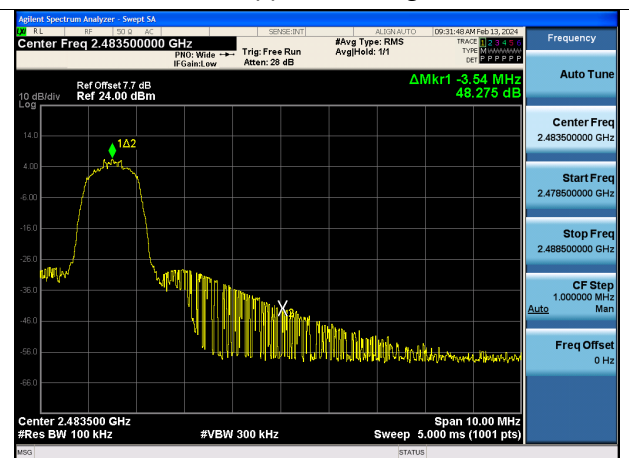
\pi/4 DQPSK Upper Band Edge(Ch. 78)
