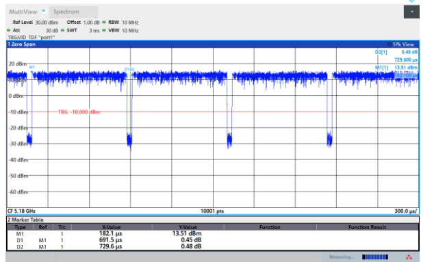
802.11ac_VHT20
