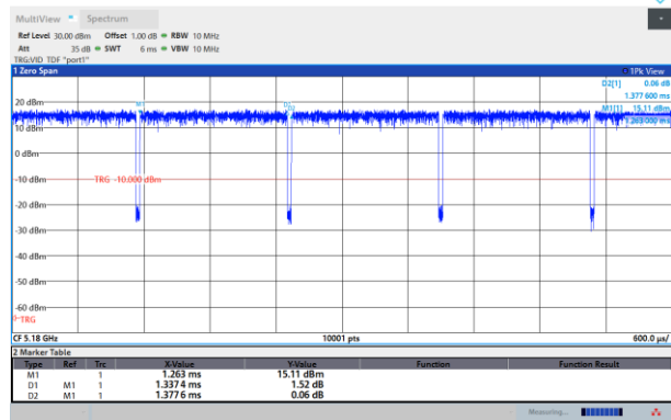
802.11ac_VHT20
