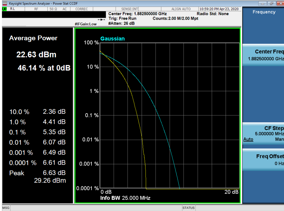
Plot 7-565. PAR Plot (Band 25/2 - 20.0MHz QPSK - Full RB Configuration)
