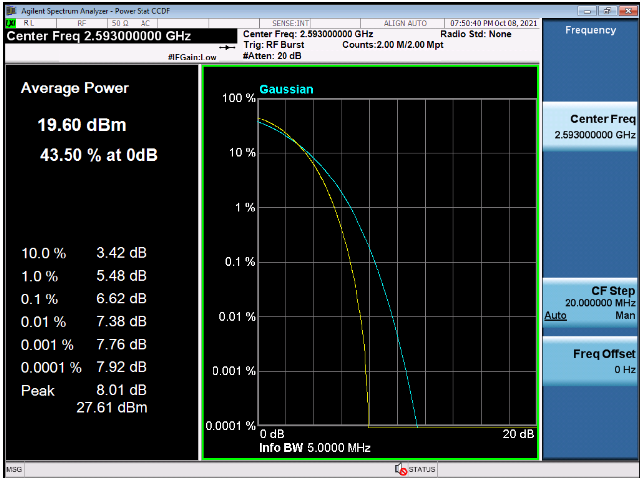
PAR Plot (5 M BW_Ch.40620_256QAM_RB25_0) (POWER CLASS 2)
