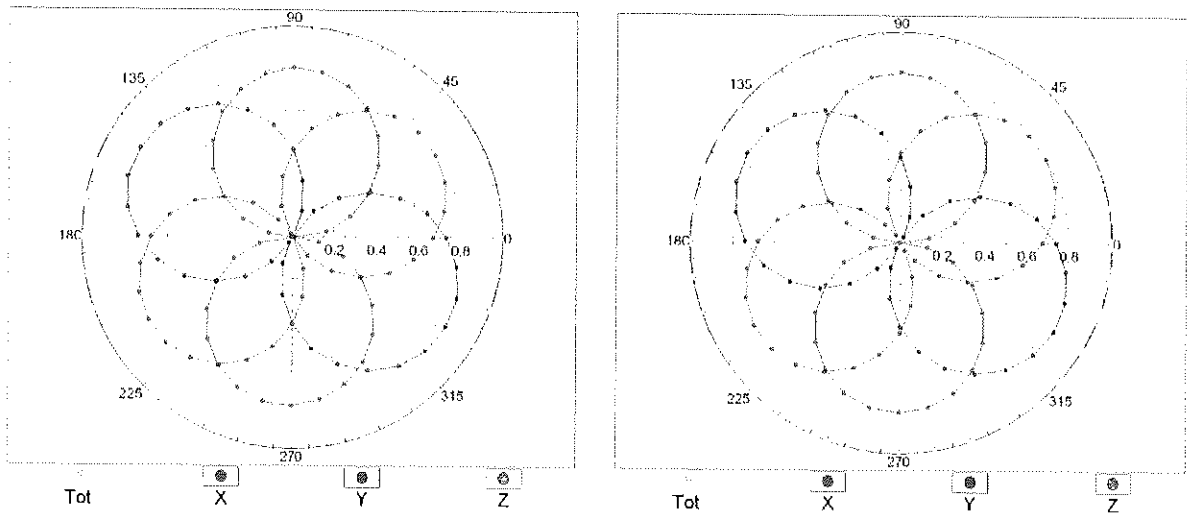
f=1800 MHz,R22
